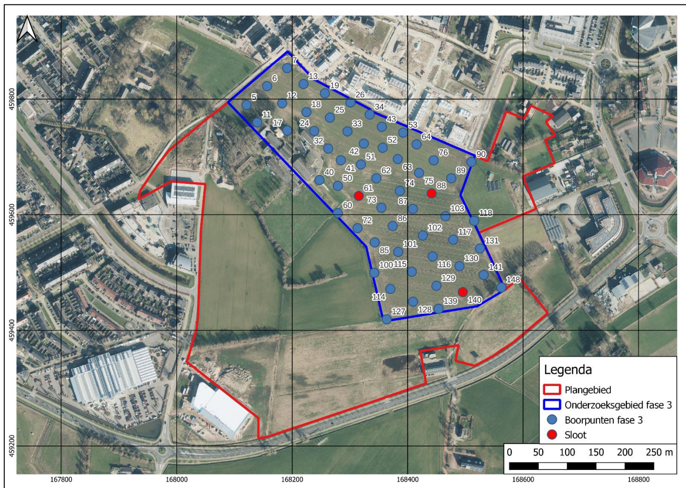
Boorpuntenkaart Fase 3
