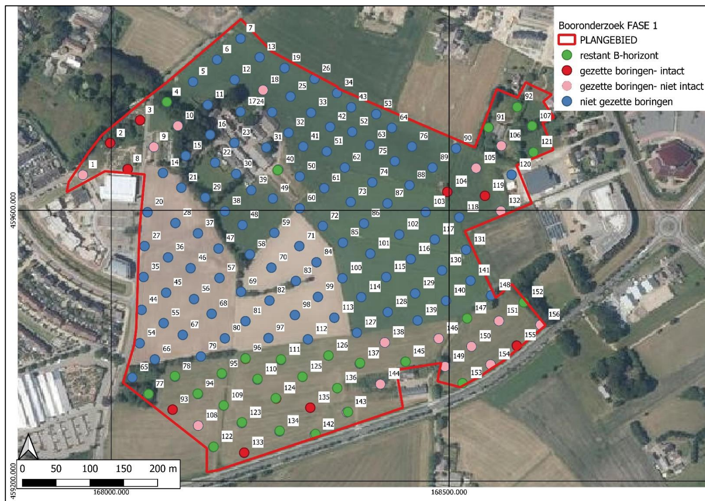
Boorpuntenkaart Fase 1
