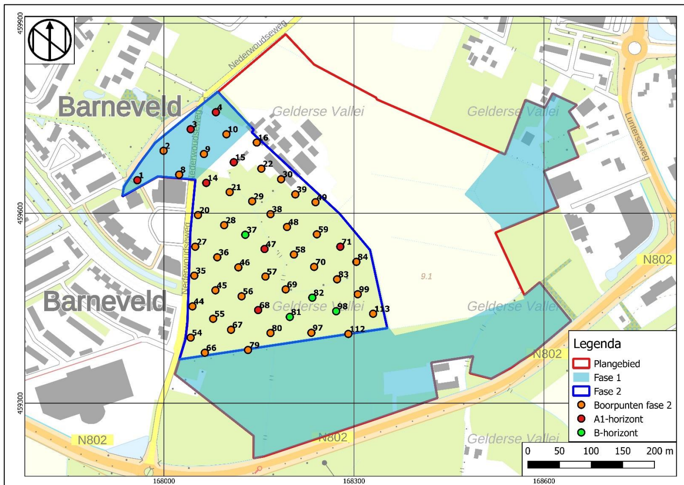
Boorpuntenkaart Fase 2
