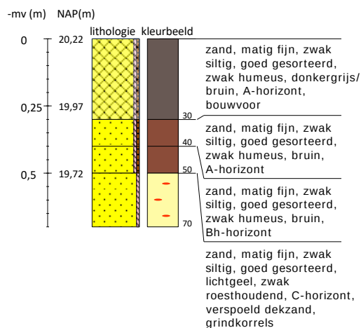
Boring 4 RD-coördinaten: 176980/462440
