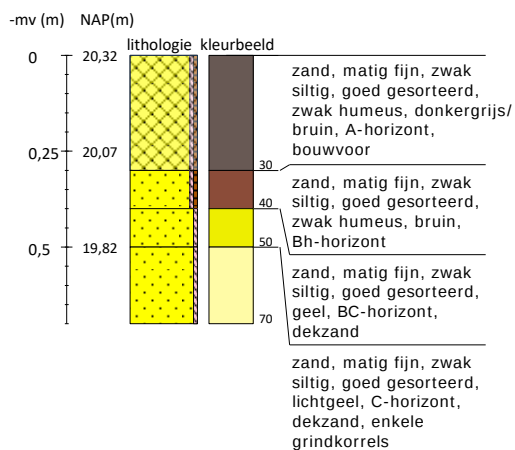
Boring 3 RD-coördinaten: 177025/462444
