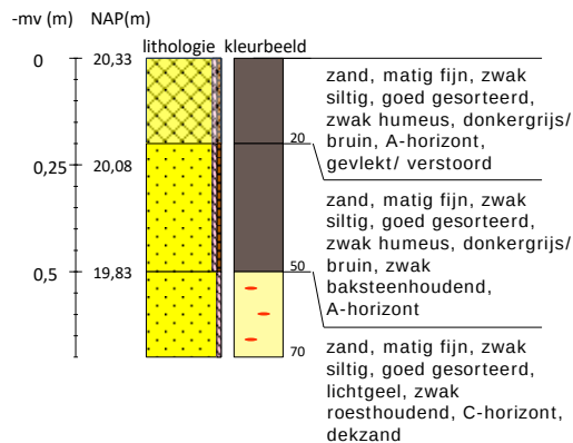
Boring 2 RD-coördinaten: 176976/462459
