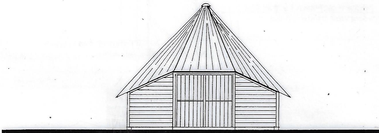
Voorgevel
