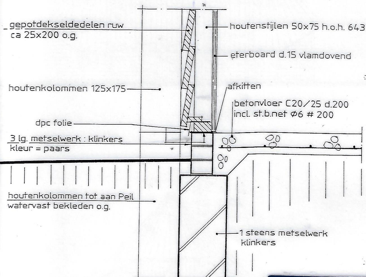
detail gevel / vloer / fundatie
