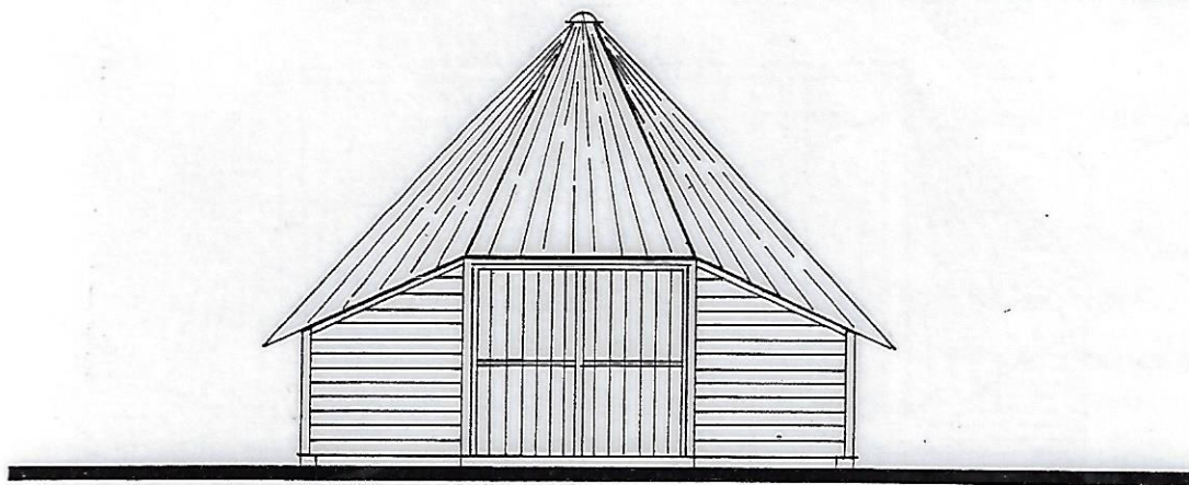
Achtergevel
