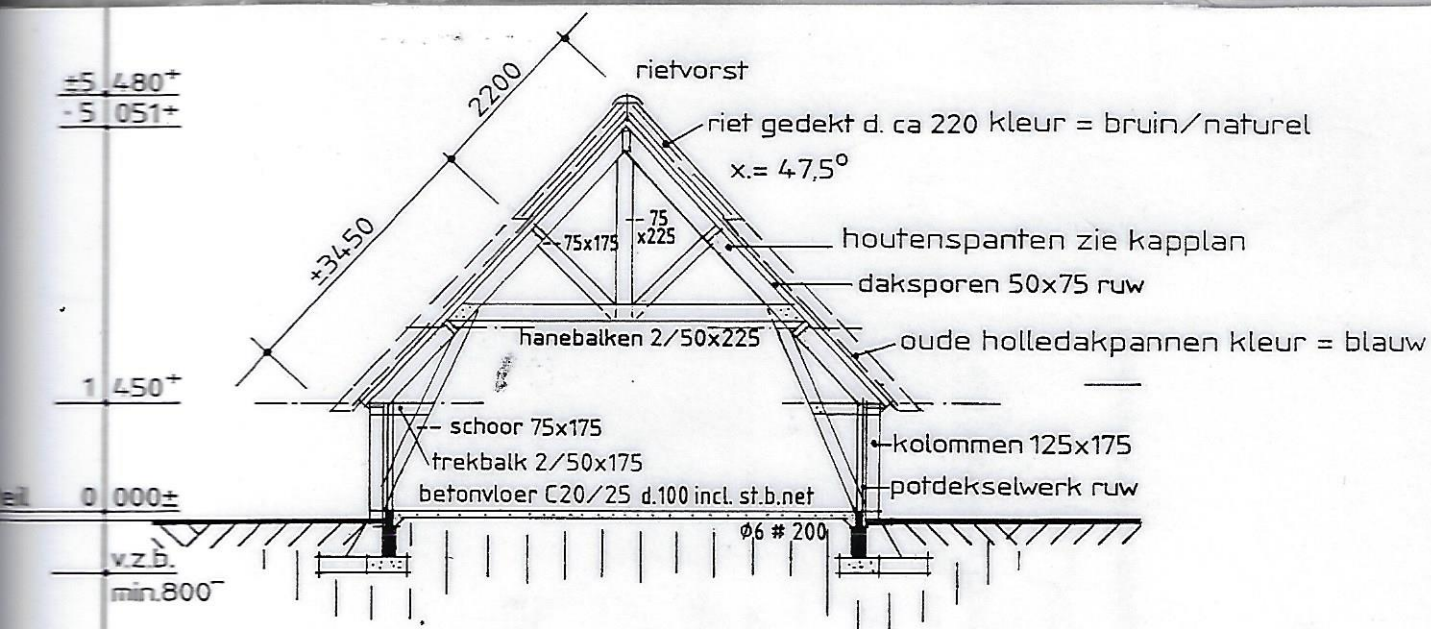
dwarsdoorsnede
