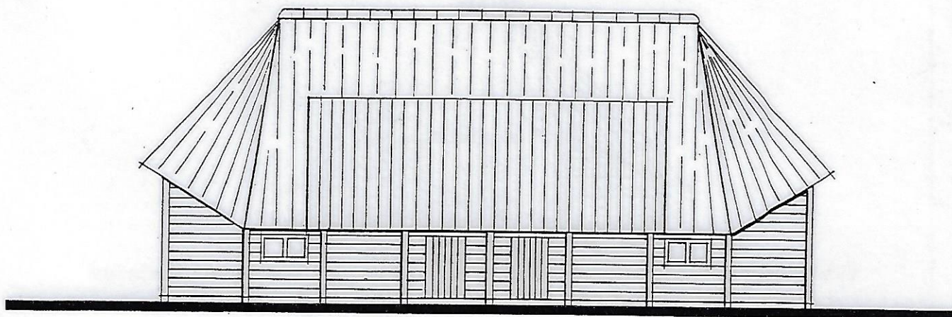
Rechterzijgevel
