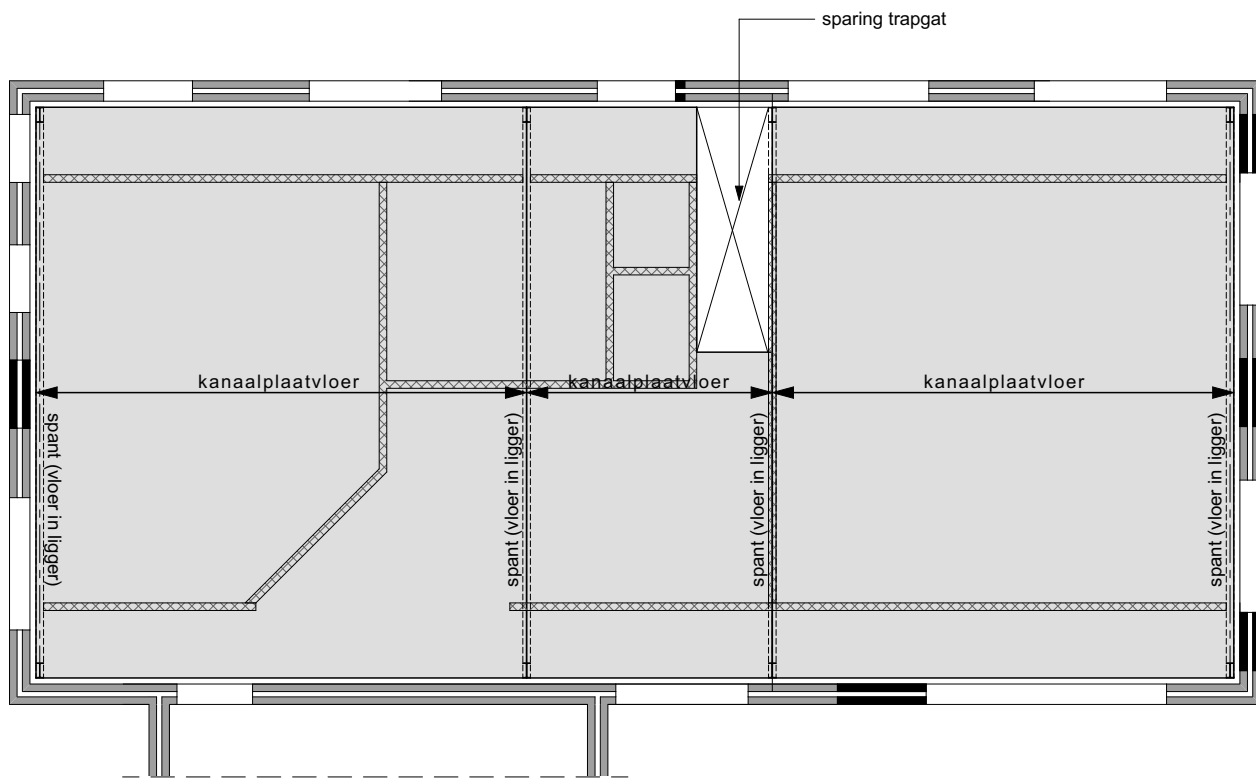
SCHEMA VERDIEPINGSVLOER
