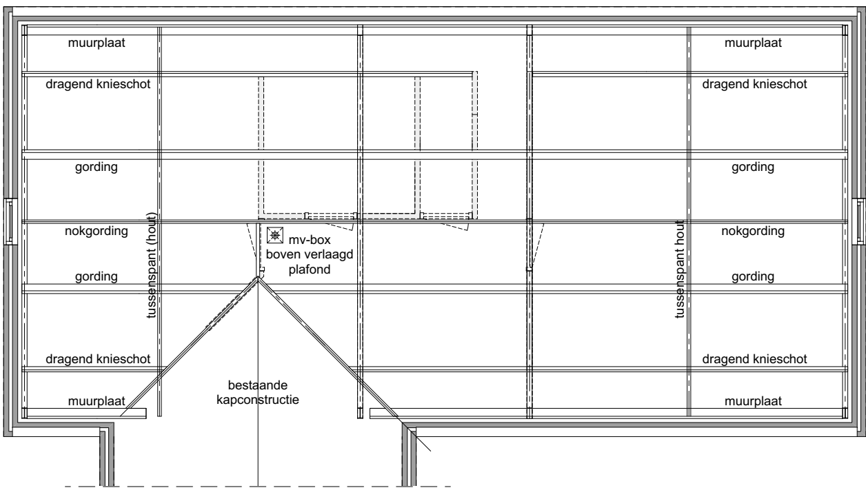
SCHEMA KAPPLAN
