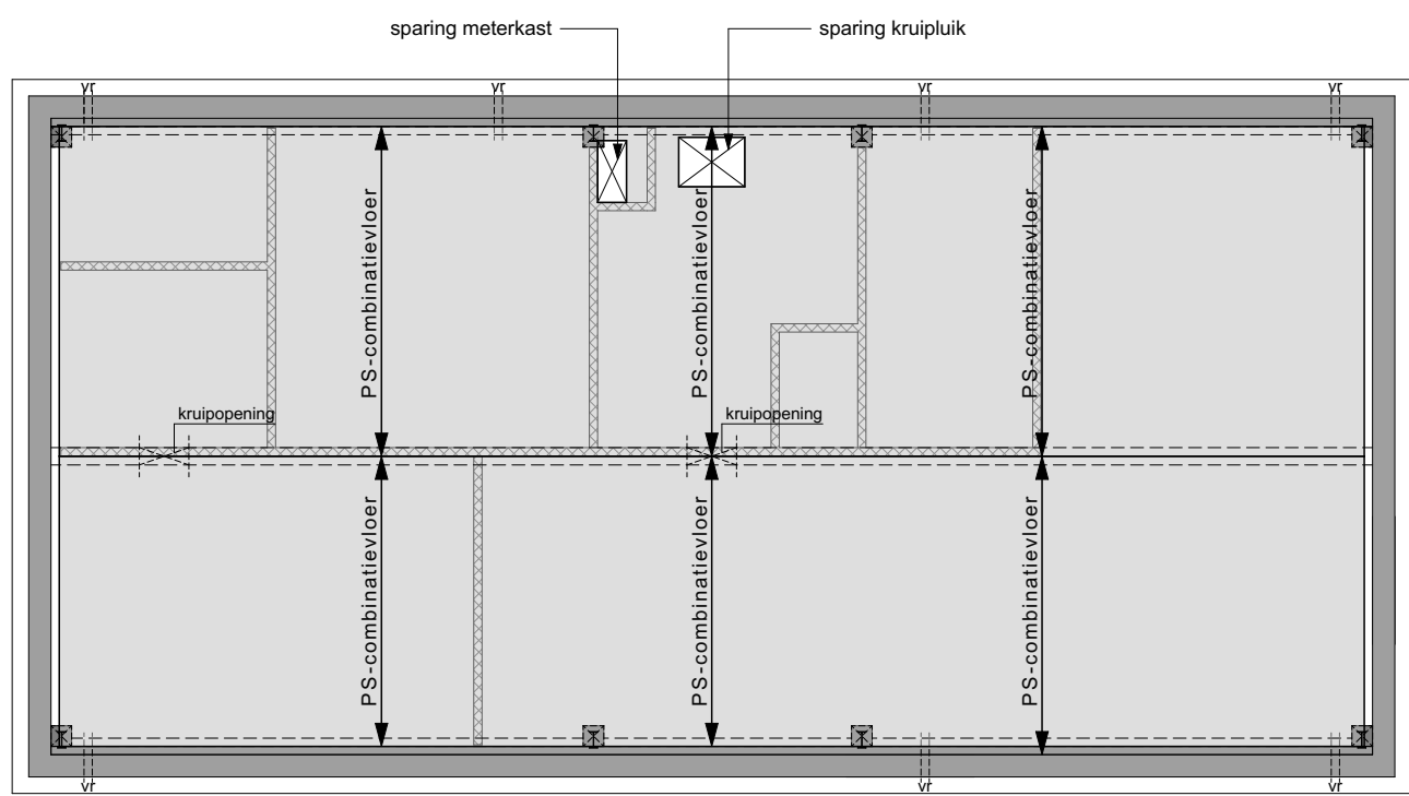
SCHEMA BEGANE GRONDVLOER
