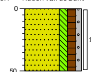
Boring: 8 Datum: 1-12-2021 Boormeester: Ruben van de Bunt
