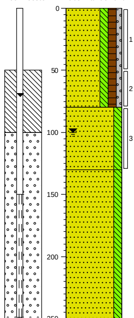
Boring: 1 Datum: 1-12-2021 Boormeester: Ruben van de Bunt
