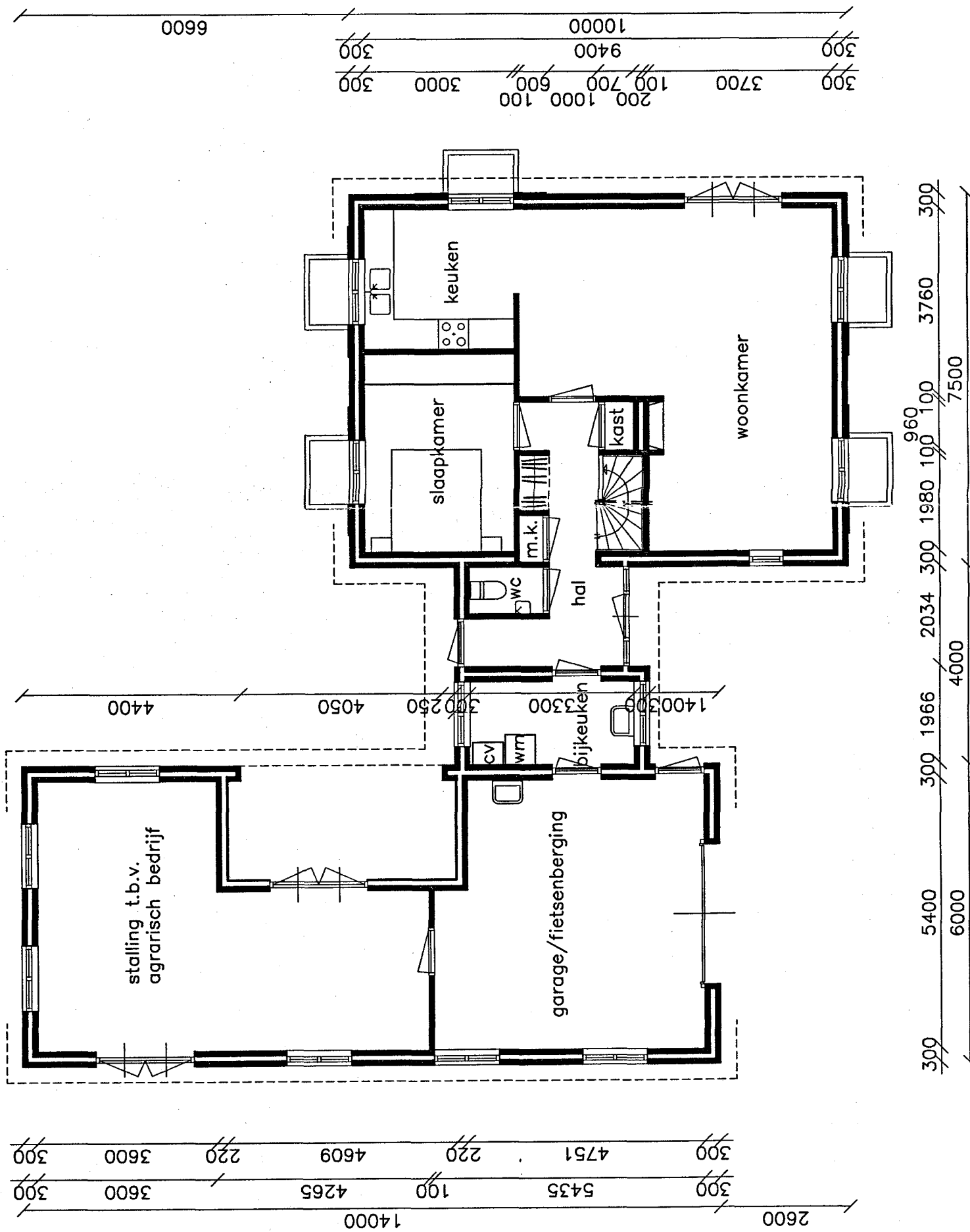
begane grond
