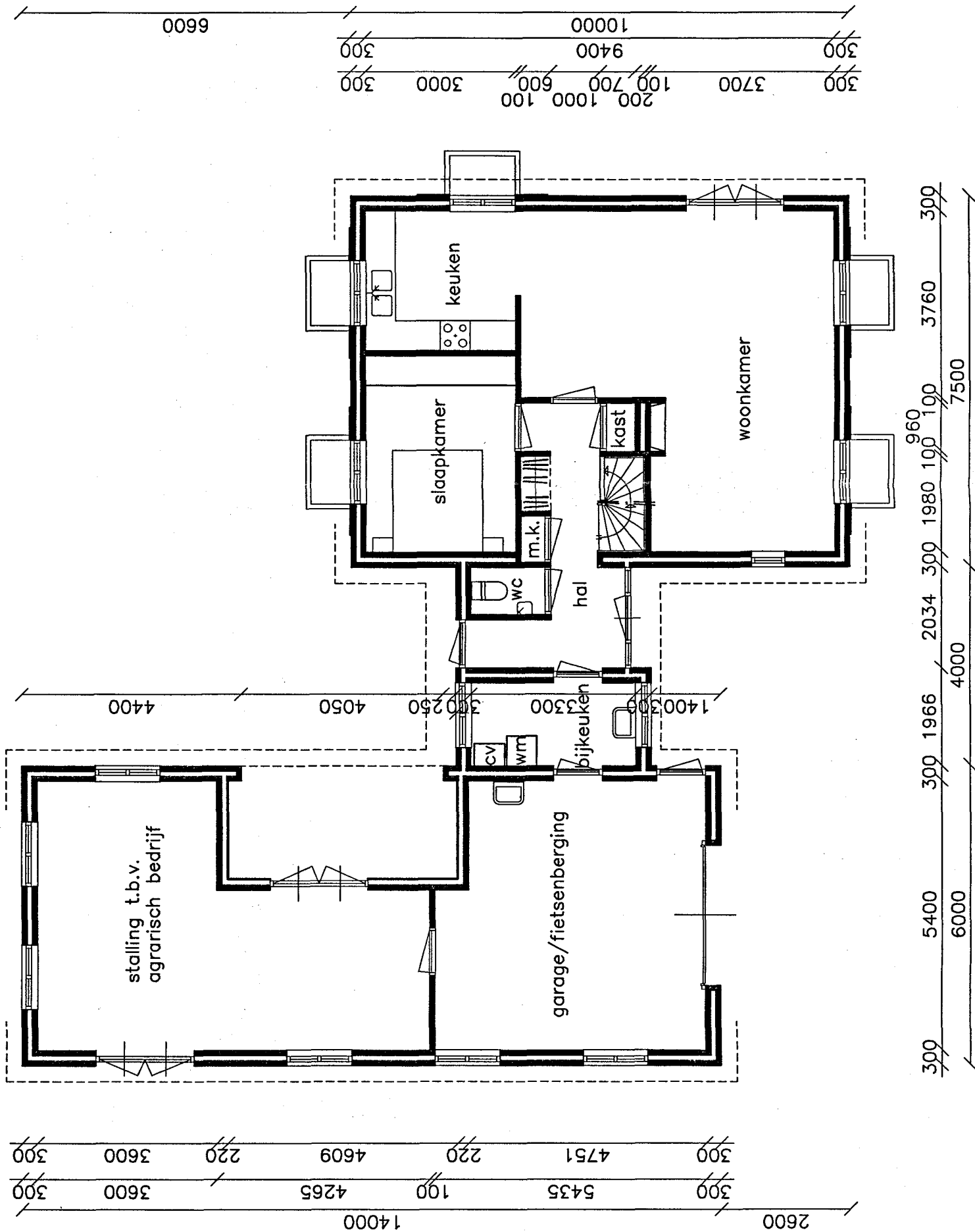
begane grond
