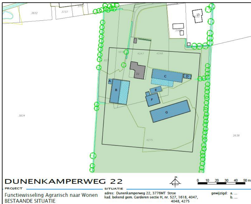
Figuur 2 Huidige inrichting van het perceel, waarbij de letters verwijzen naar de opsomming onder planlocatie . De blauwe opstallen worden gesaneerd in de beoogde ingreep (bron: dbl architectenbureau).
