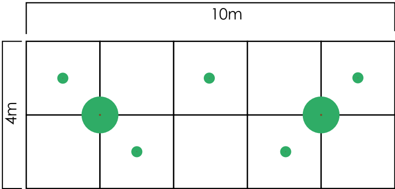
Principeschets plantverband houtwal
