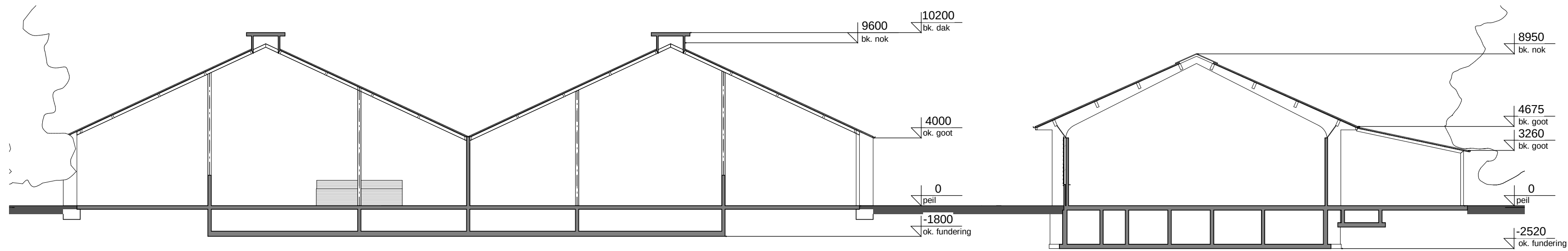
Doorsnede A-A
