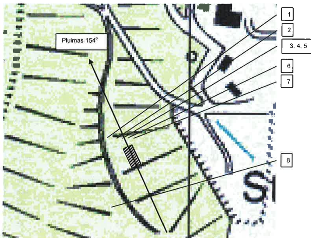
Figuur 5.1.3. Meetposities op het stortvak tijdens meetserie 1
