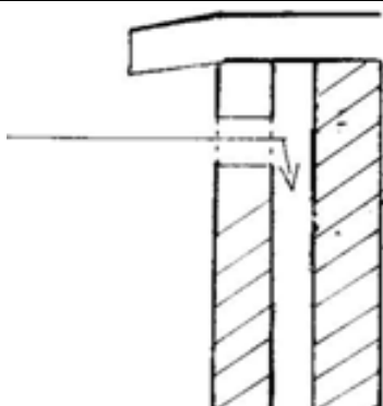
Figuur 2.1 Invliegopening in spouwmuur: breedte invliegopening maximaal 2 cm
