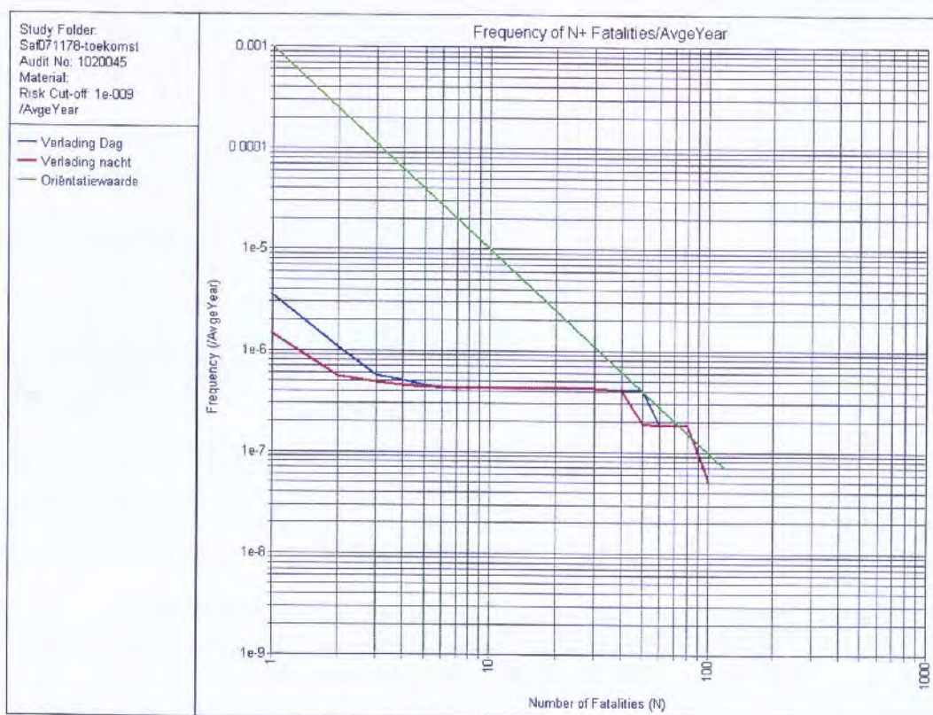
Figuur 4. Groepsrisico LPG-tankstation toekomstige situatie bevoorrading overdag en 's avonds
