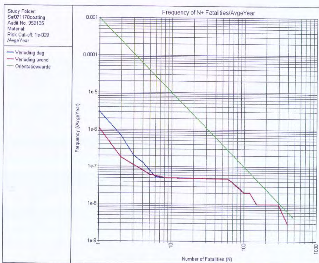
Figuur 5. Groepsrisico LPG-tankstation bevoorrading overdag en 's avonds (tankauto voorzien van een hittewerende coating)
