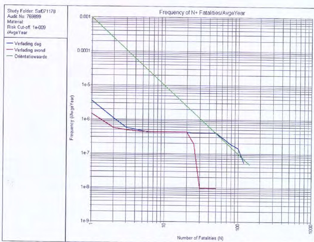
Figuur 3. Groepsrisico LPG-tankstation huidige situatie bevoorrading overdag en 's avonds
