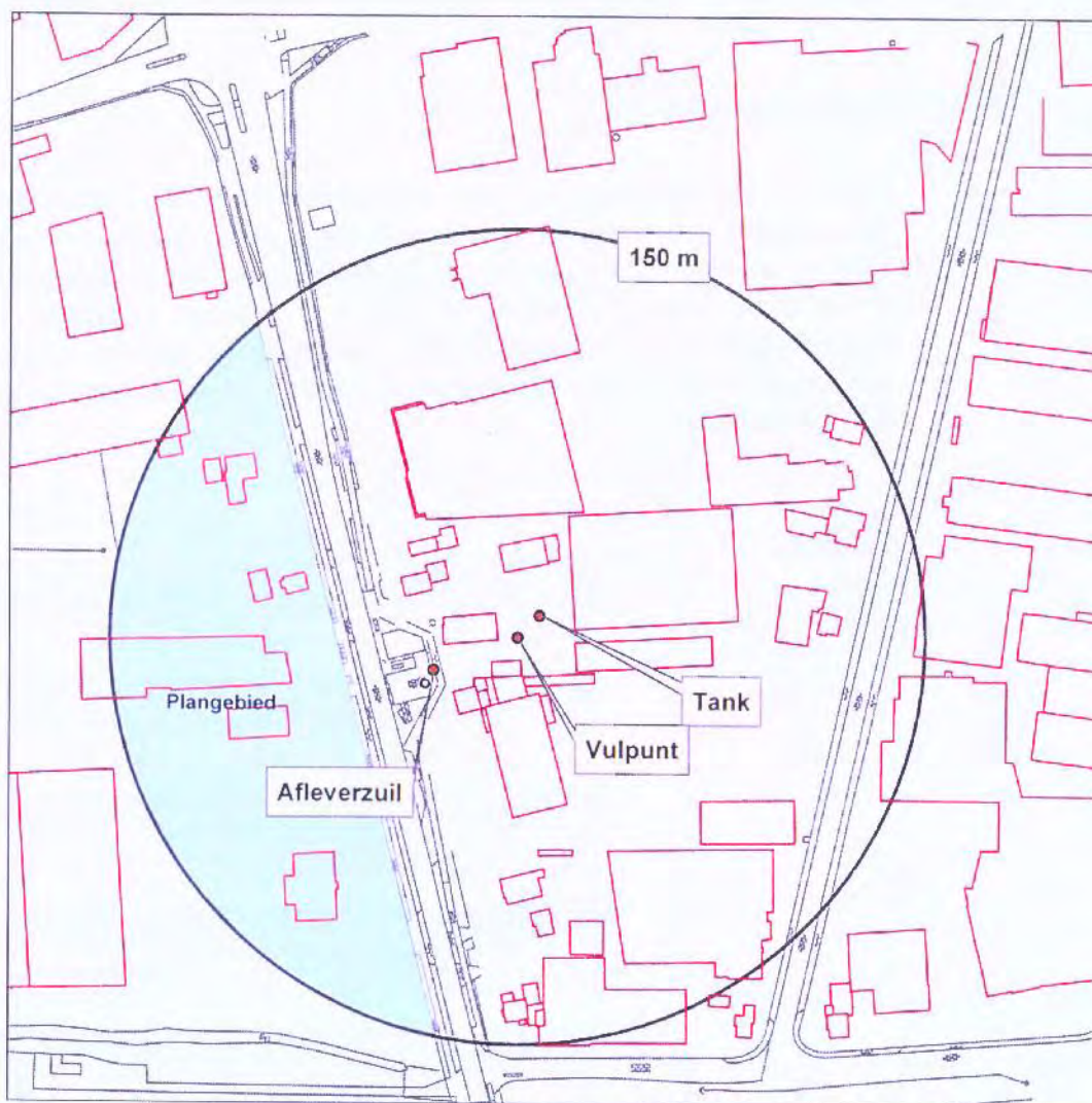
Figuur 2. Plangebied binnen invloedsgebied LPG-tankstation
