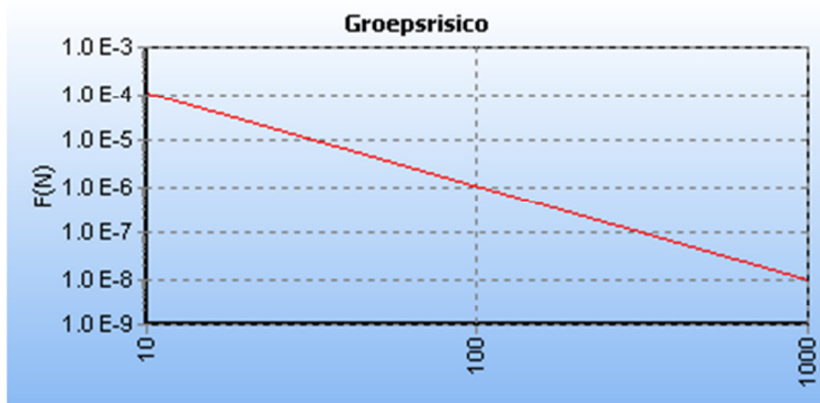
5.5 Figuur 5.5 FN curve voor N-571-81 van N.V. Nederlandse Gasunie voor de kilometer tussen stationing 2390.00 en stationing 3390.00
