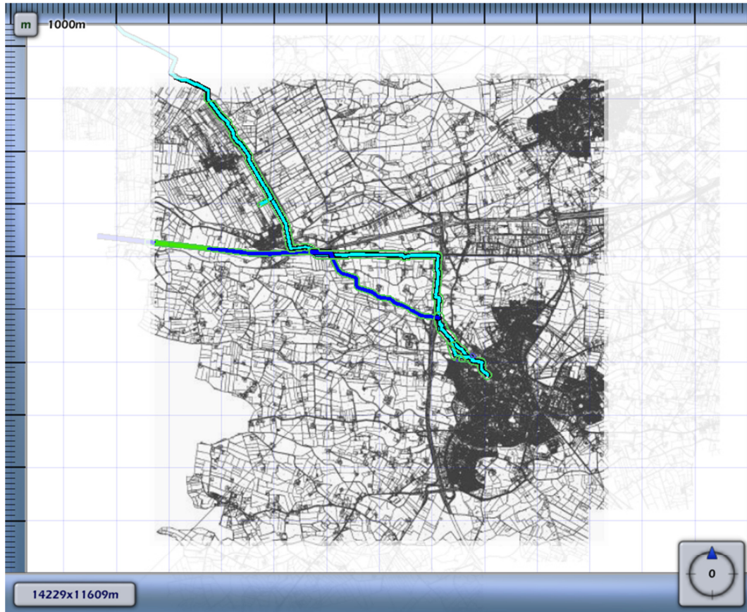
Figuur 4.10 Kilometer leiding behorende bij de maximale overschrijding van de FN-curve voor N-571-81 van N.V. Nederlandse Gasunie
