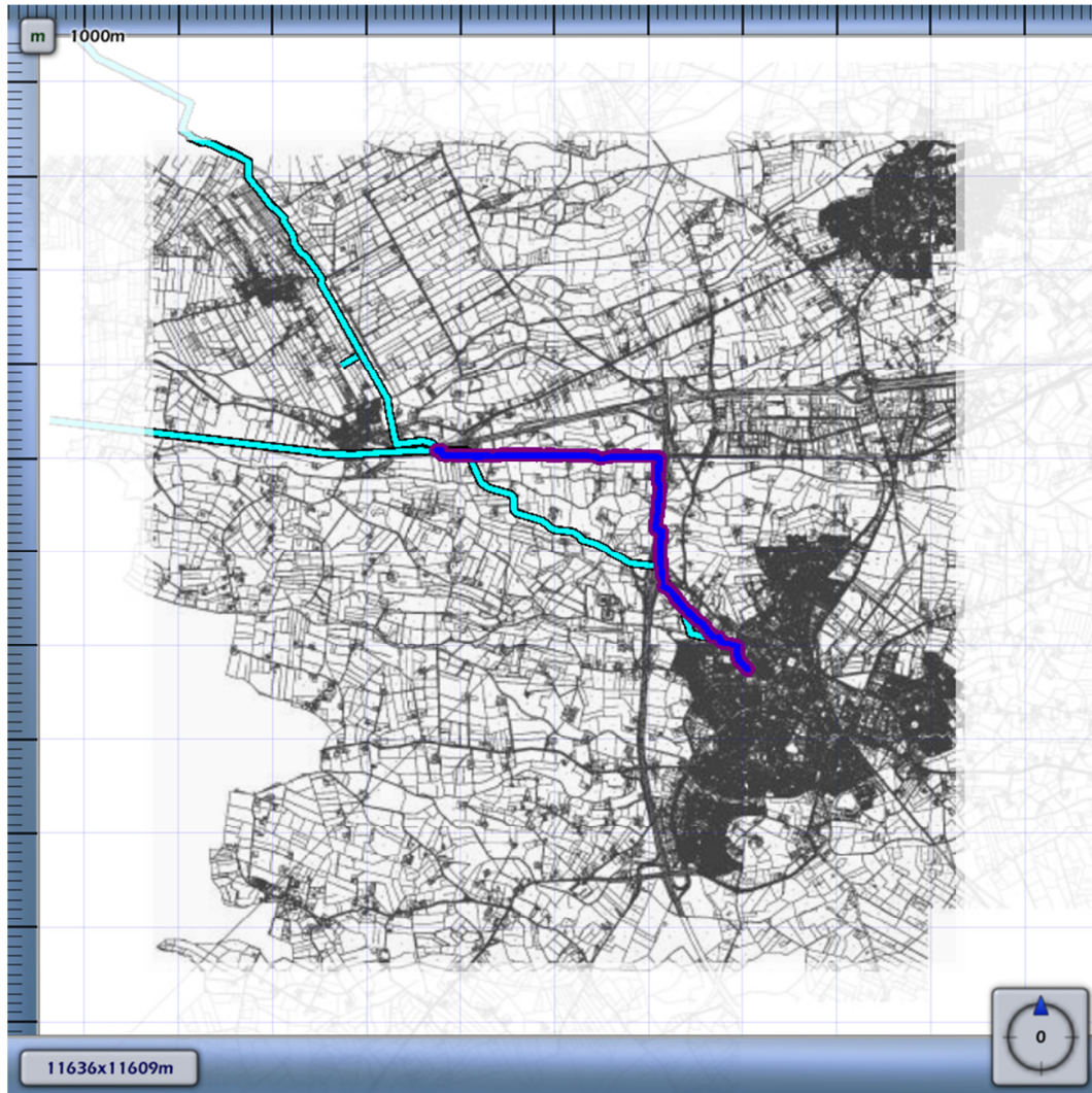
3.1 Figuur 3.1 Plaatsgebonden risico voor N-570-38 van N.V. Nederlandse Gasunie
