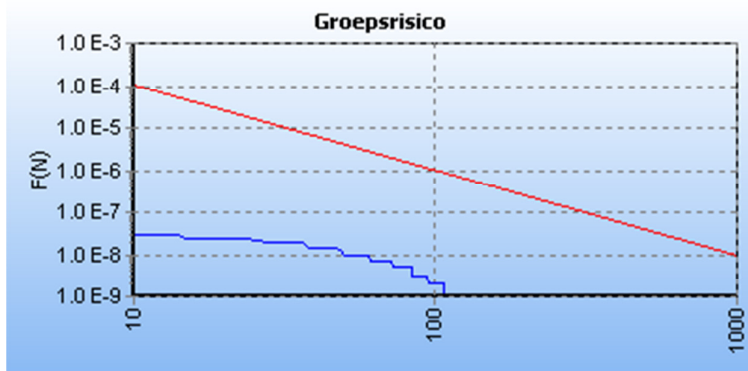
5.4 Figuur 5.4 FN curve voor N-570-44 van N.V. Nederlandse Gasunie voor de kilometer tussen stationing 0.00 en stationing 1000.00
