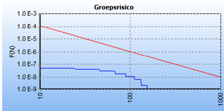
5.2 Figuur 5.2 FN curve voor N-570-39 van N.V. Nederlandse Gasunie voor de kilometer tussen stationing 2360.00 en stationing 3360.00
