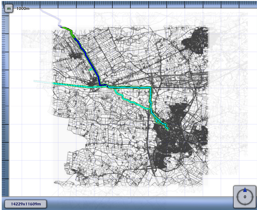
Figuur 4.4 Kilometer leiding behorende bij de maximale overschrijding van de FN-curve voor N-570-39 van N.V. Nederlandse Gasunie
