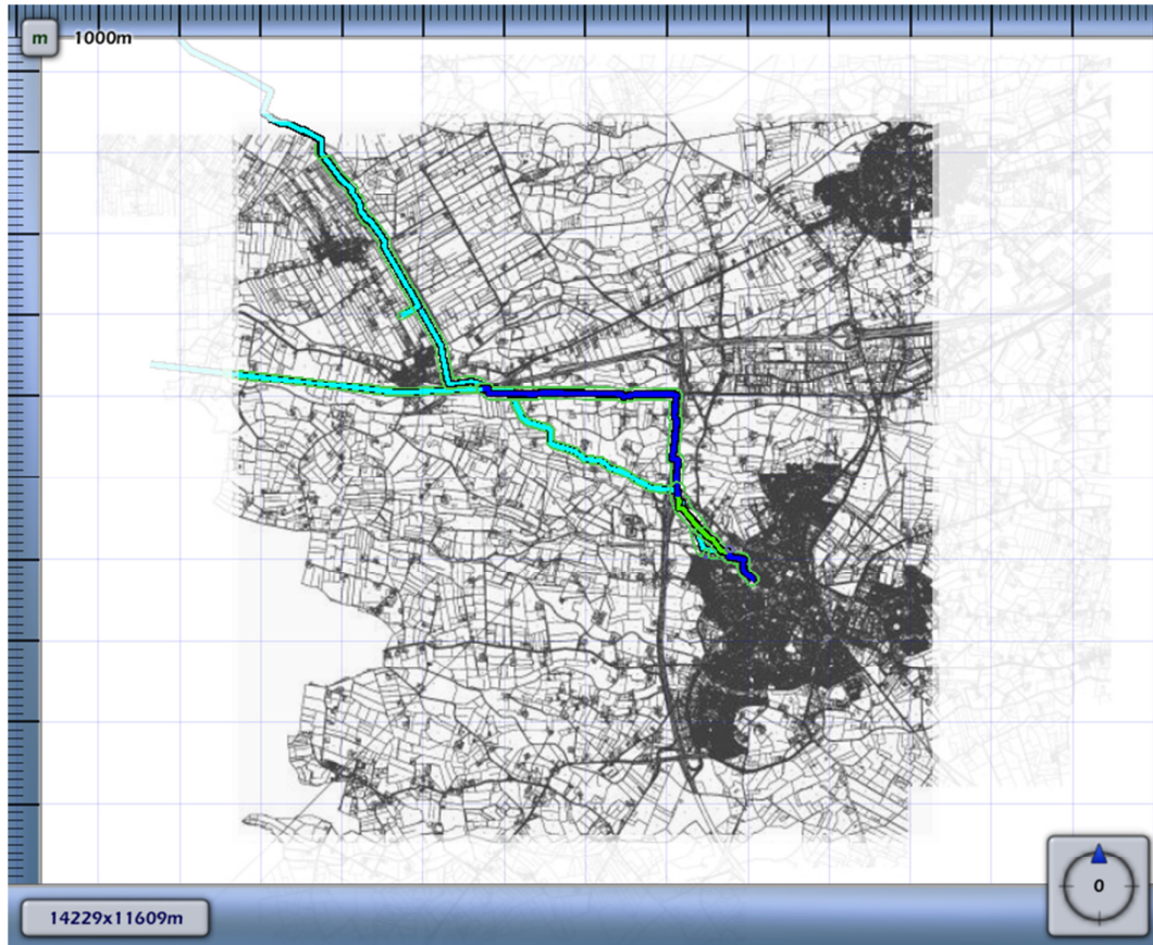
Figuur 4.2 Kilometer leiding behorende bij de maximale overschrijding van de FN-curve voor N-570-38 van N.V. Nederlandse Gasunie
