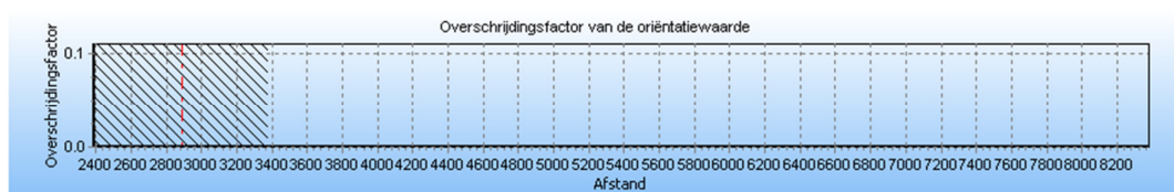
4.5 Figuur 4.9 Groepsrisico screening voor N-571-81 van N.V. Nederlandse Gasunie
