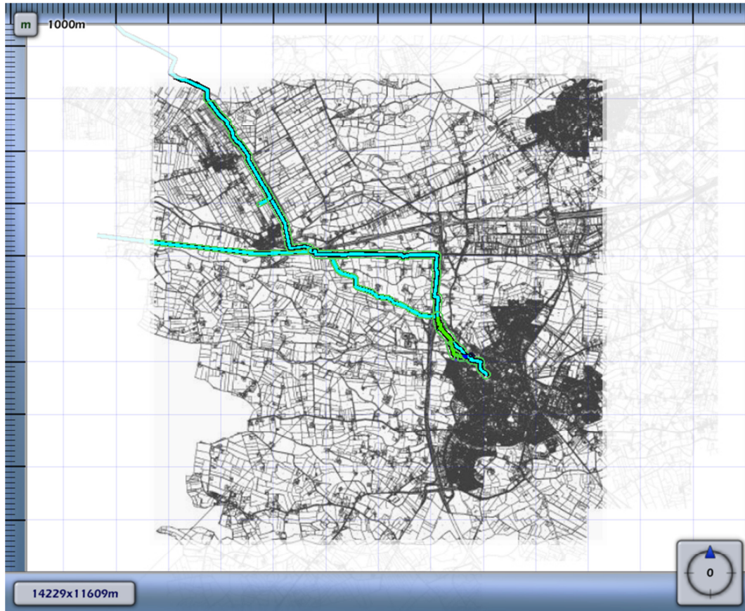
Figuur 4.8 Kilometer leiding behorende bij de maximale overschrijding van de FN-curve voor N-570-44 van N.V. Nederlandse Gasunie
