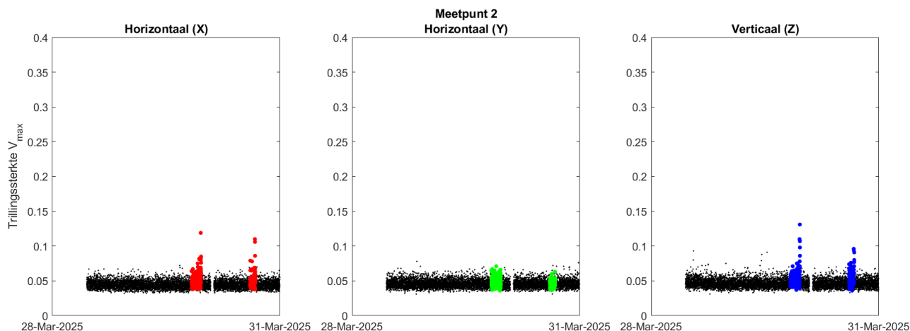
Figuur 75 Gemeten trillingen bij meetpunt 2 (maaiveld hoek Pleijweg-Nijmeegseweg)
