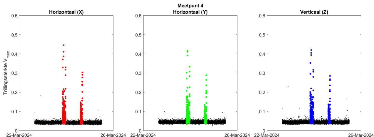
Figuur 51 Gemeten trillingen bij meetpunt 4 (maaiveld bij winkelcentrum)
