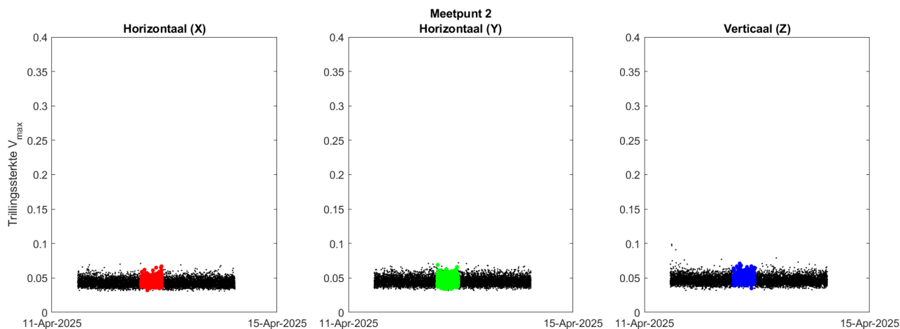
Figuur 90 Gemeten trillingen bij meetpunt 2 (maaveld hoek Pleijweg-Nijmeegseweg)
