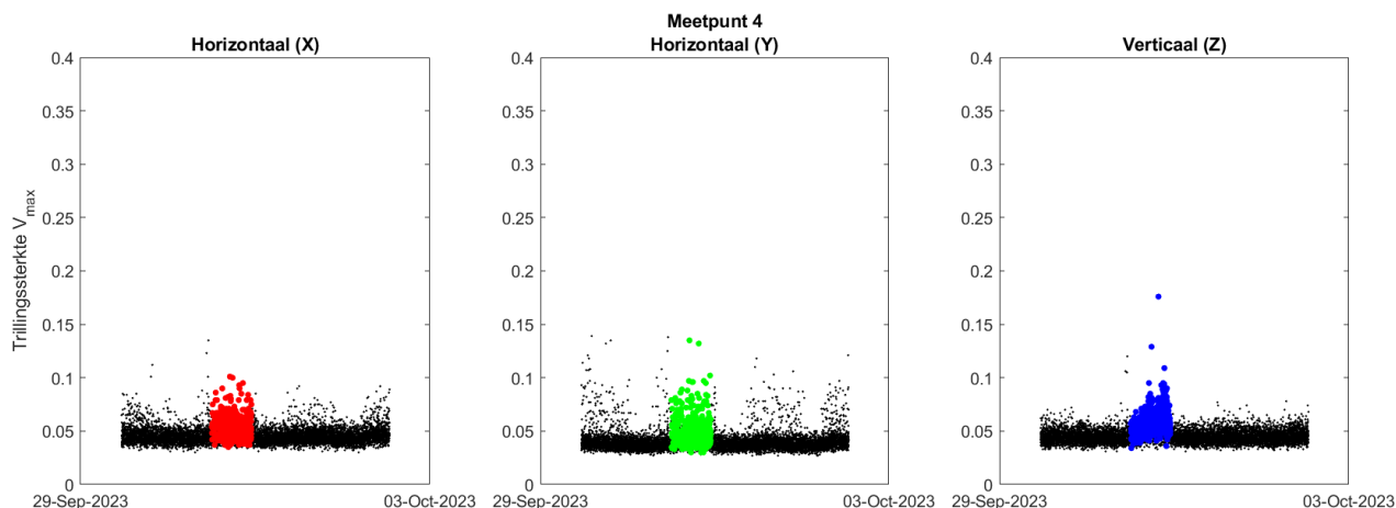
Figuur 18 Gemeten trillingen bij meetpunt 4 (maaiveld Batavierenweg - Nijmeegseweg)
