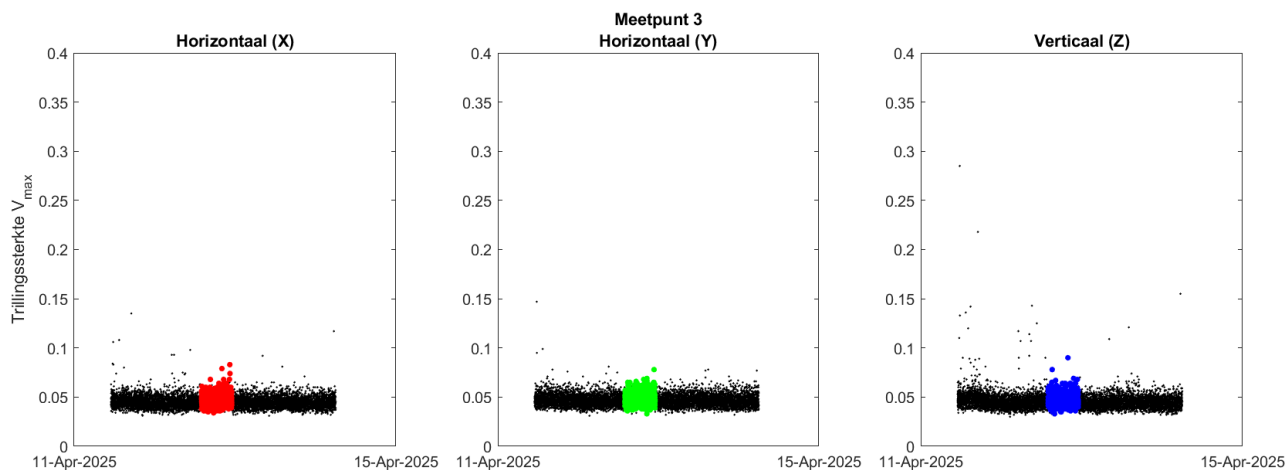
Figuur 93 Gemeten trillingen bij meetpunt 3 (maaiveld Schepen ten Havestraat)
