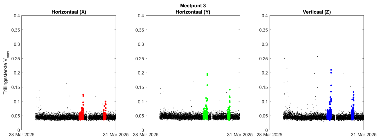
Figuur 78 Gemeten trillingen bij meetpunt 3 (maaiveld Schepen ten Havestraat)
