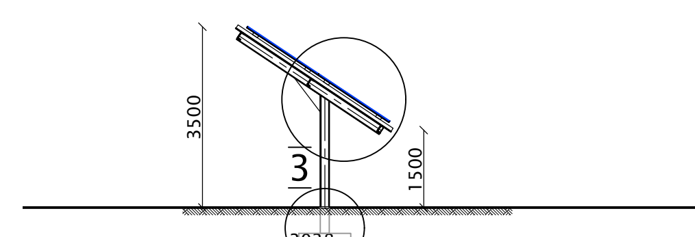
plek B: frame langs jeugdbaan, bedekt met 160st. PV-panelen, schaal 1:200
