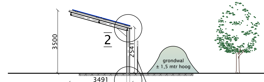
plek A: frame langs erfgrns, bedekt met 100st. PV-panelen, schaal 1:200
