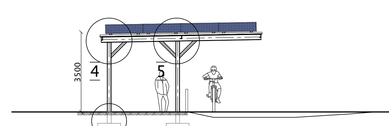
plek C: frame langs baan, bedekt met 240 st. PV-panelen, schaal 1:200
