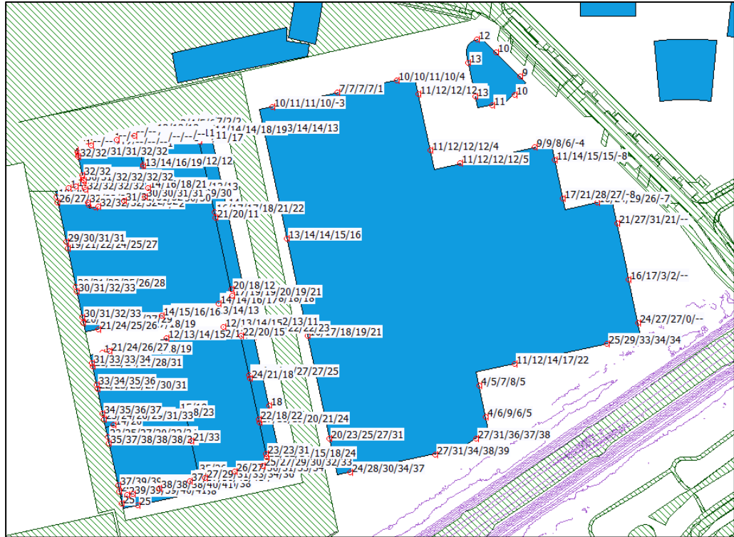
Figuur 8 Berekende geluidbelasting per toetspunt ten gevolge van de gezoneerde Merwedestraat inclusief aftrek conform artikel 110g Wgh
