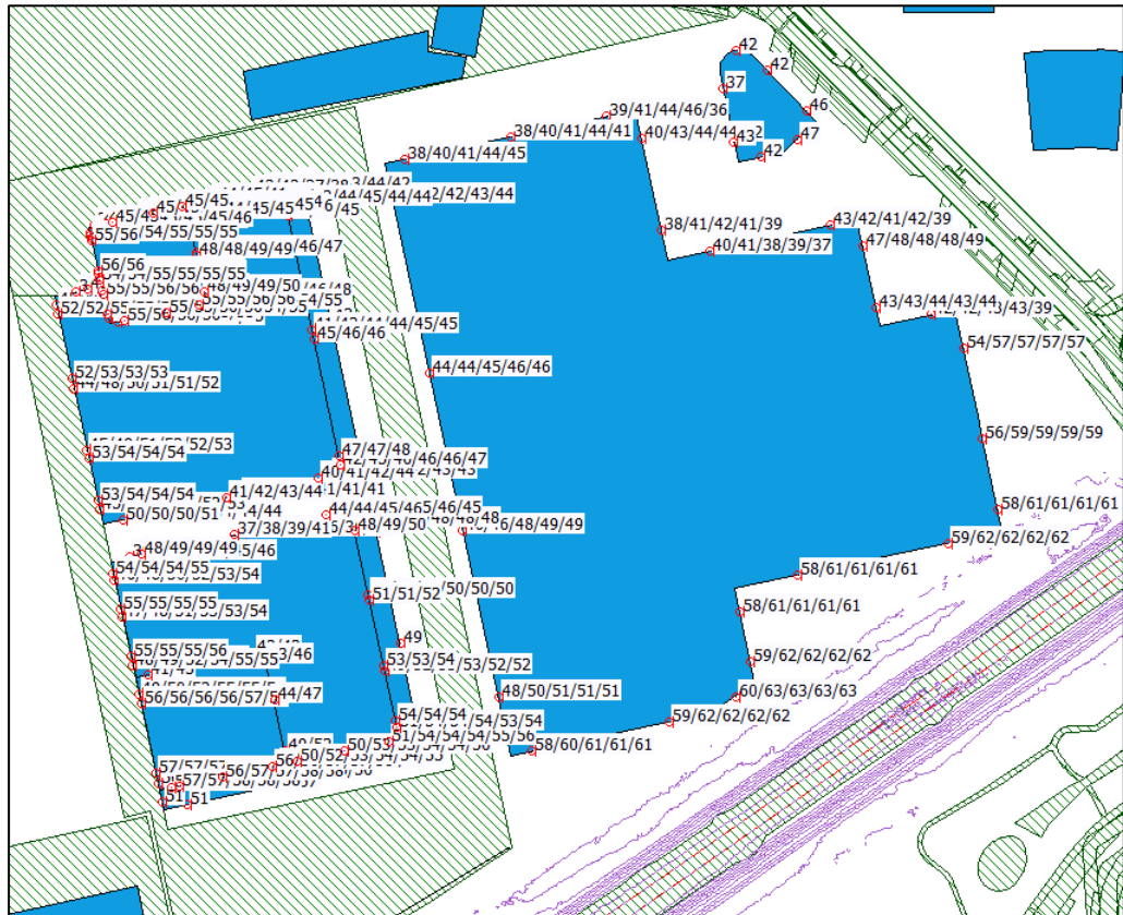
Figuur 6 Berekende geluidbelasting per toetspunt ten gevolge van de gezoneerde spoorlijnen
