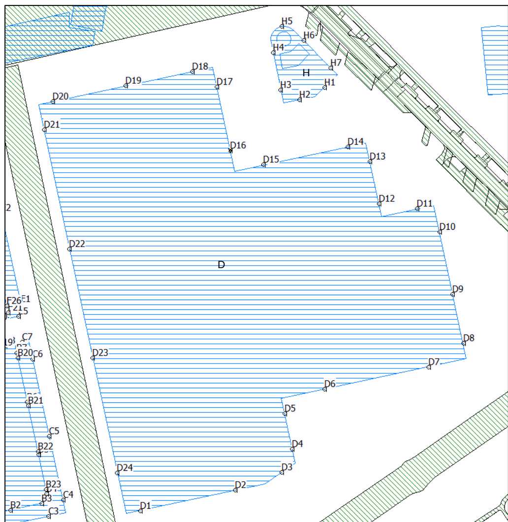
Figuur 4A.2 Ligging toetspunten gebied D en H (maximale planologische mogelijkheden)
