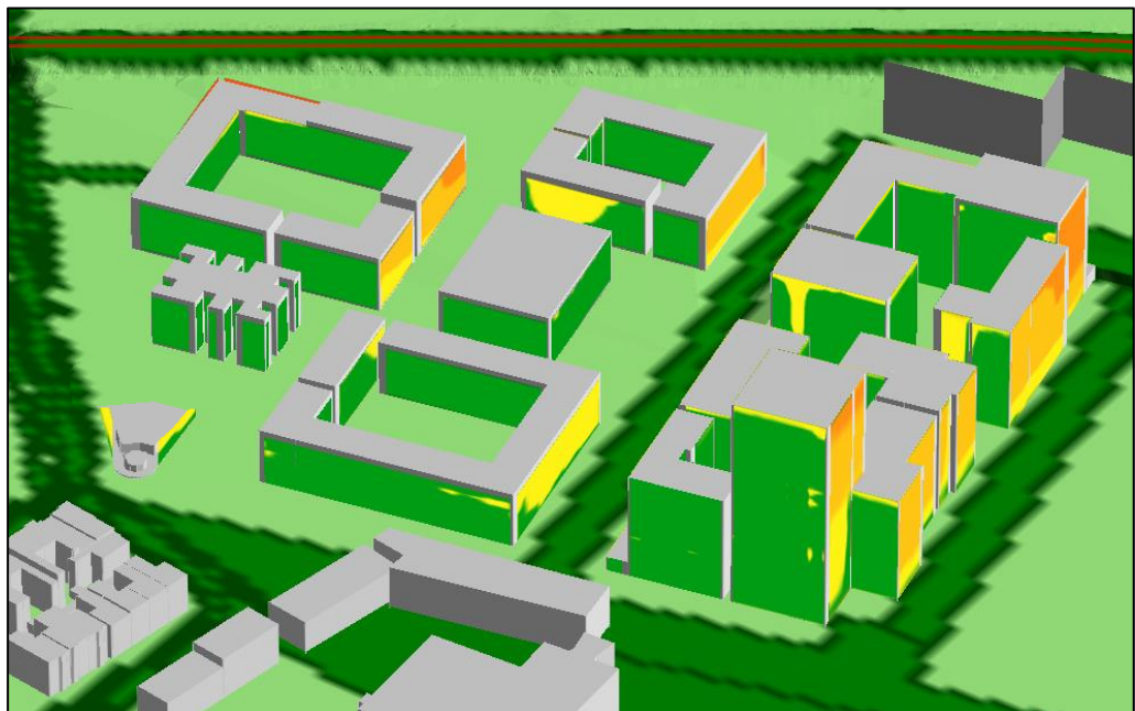
Figuur 11C Gekleurde 3D-weergave berekende geluidbelasting noordzijde railverkeerslawaaï
