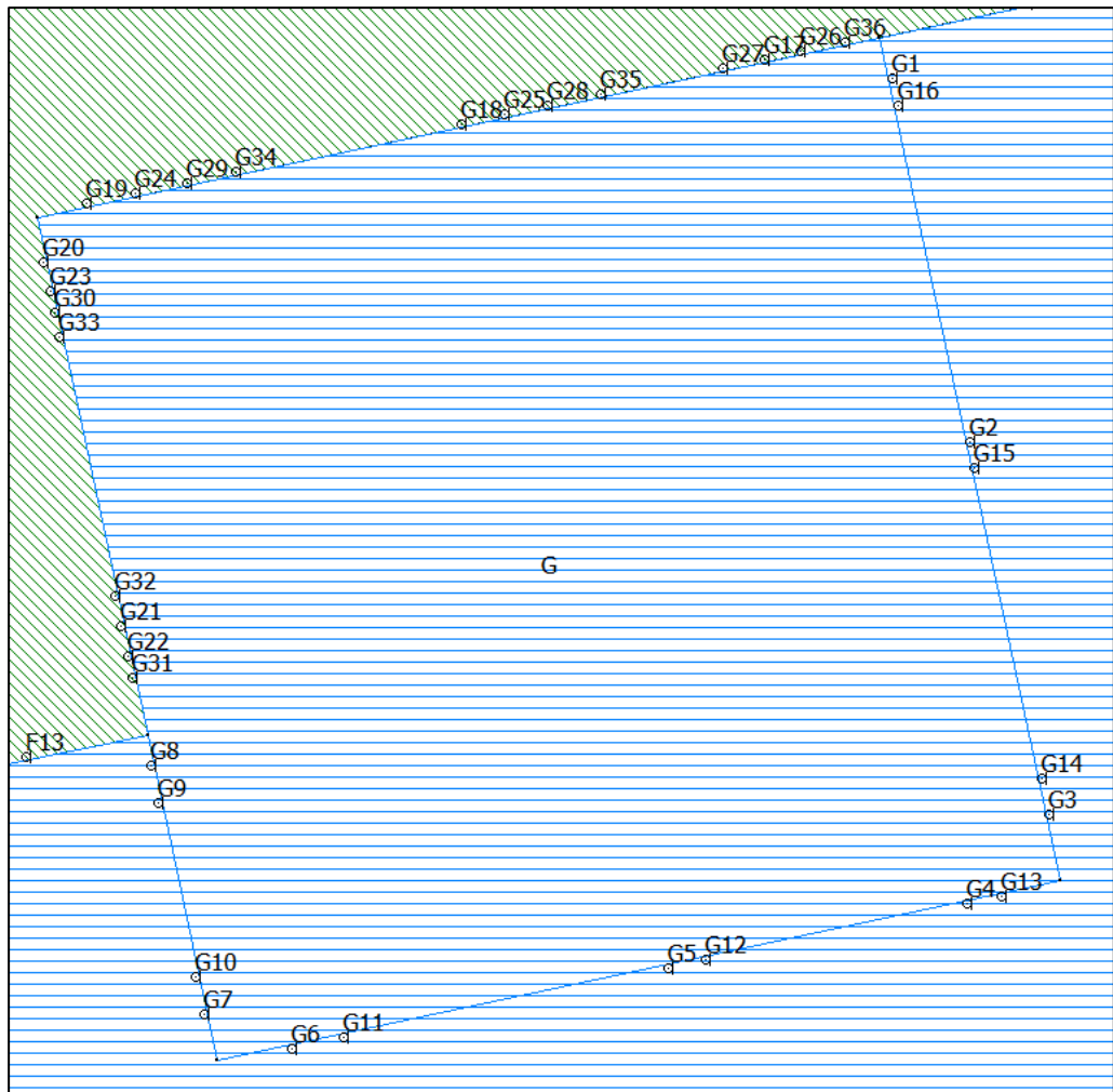
Figuur 4A.4 Ligging toetspunten gebouw G (maximale planologische mogelijkheden)
