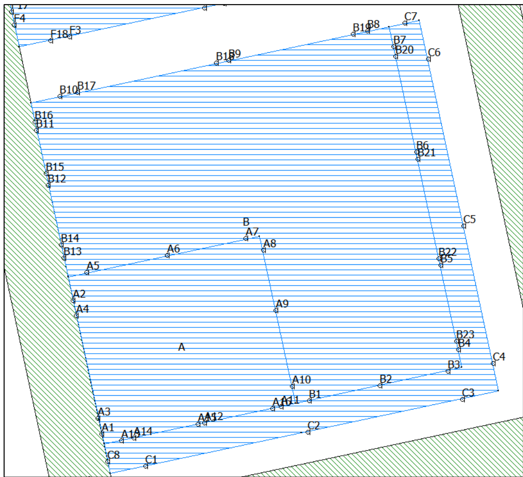
Figuur 4A.1 Ligging toetspunten gebouw A-C (maximale planologische mogelijkheden)
