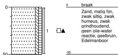
Boring: 5 boormeester j molenkamp Sleuflengte [m]: 0,00 Sleufbreedte [m]: 0,00
