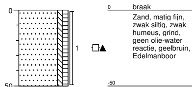
Boring: 2 boormeester j molenkamp Sleuflengte [m]: 0,00 Sleufbreedte [m]: 0,00
