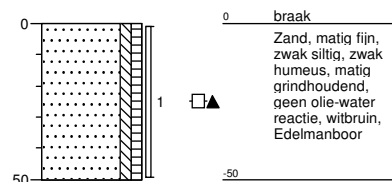
Boring: 6 boormeester j molenkamp Sleuflengte [m]: 0,00 Sleufbreedte [m]: 0,00
