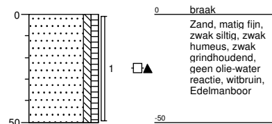
Boring: 3 boormeester j molenkamp Sleuflengte [m]: 0,00 Sleufbreedte [m]: 0,00
