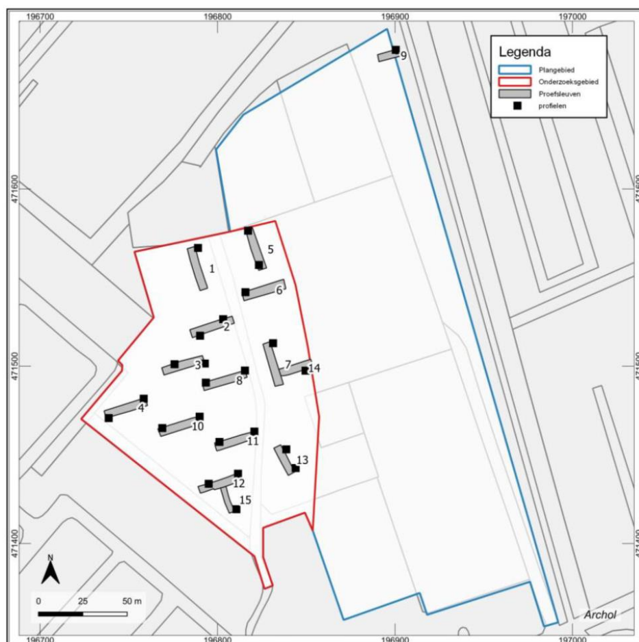
Figuur 2: het plangebied en het onderzoeksgebied met de aangelegde proefsleuven en profielen (bron: Brattinga, 2025).
