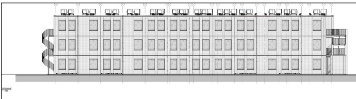
Afbeelding 2.3 Impressie voorgevel westelijk gebouw (Bron: Plegt-Vos Bouwgroep)
