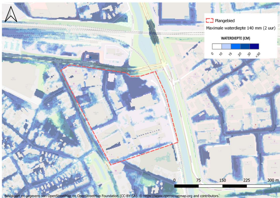
Afbeelding 3.16 Risico op wateroverlast bij extreme neerslag (bron: RIVM, 2018)
