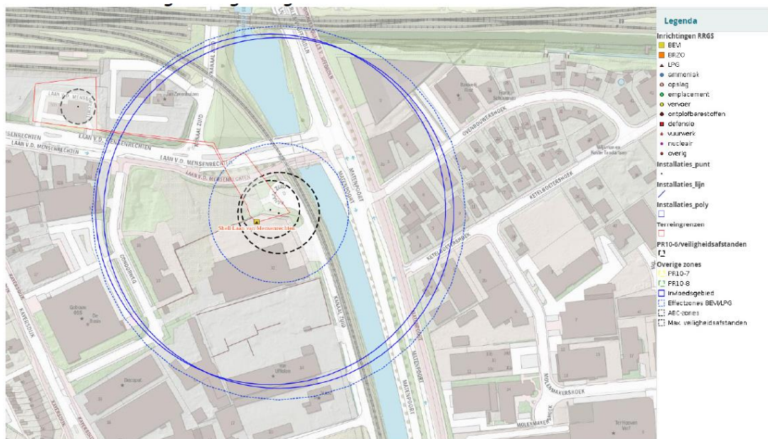
Afbeelding 3.10 Verkooppunt voor motorbrandstoffen met 10^{-6} contour (zwarte stippellijn) en invloedsgebied (blauwe lijn)
