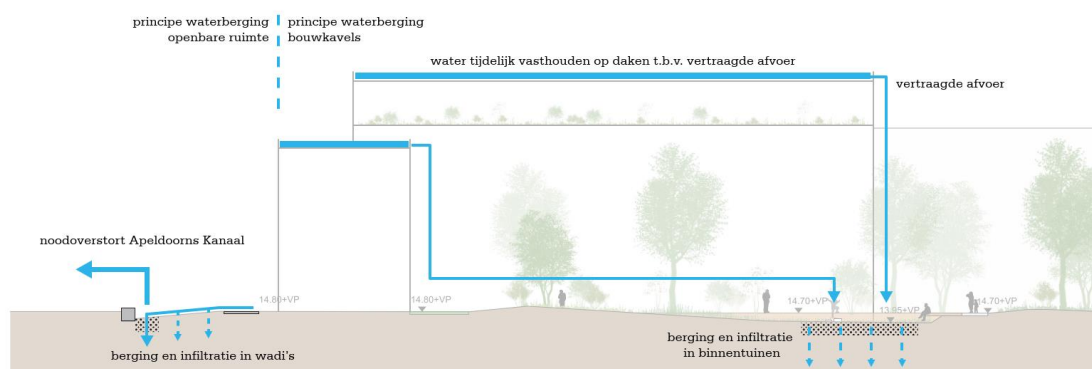
Afbeelding 4.11 maatregelen voor waterberging (bron: Rijnboutt, 2021)
