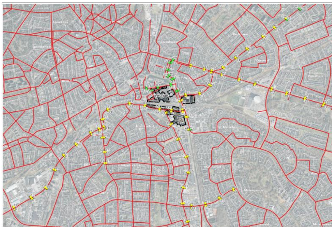
Afbeelding 3.1 Verschil \text{NO}_2 -concentraties 2030 - situatie raakvlakproject Spoorzone Oost met Kayersmolen-Noord
