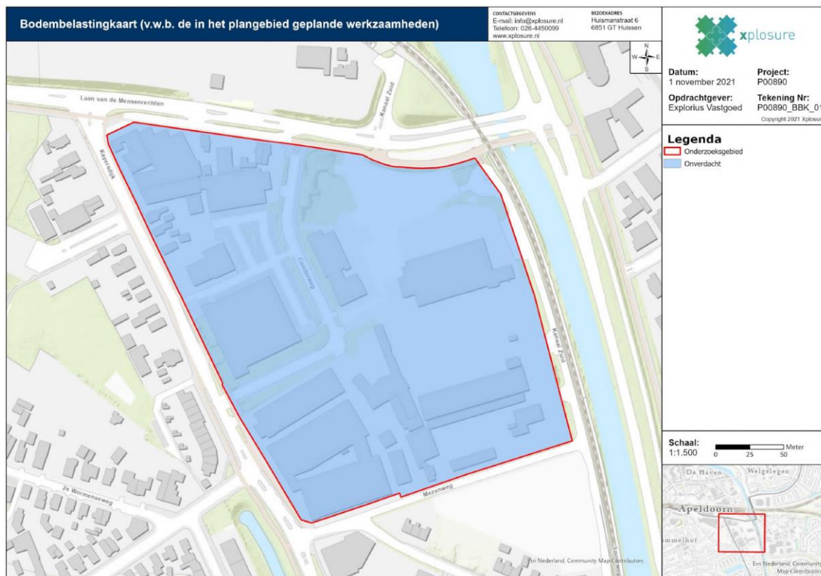
Afbeelding 3.14 Bodembelastingkaart (bron: Xplosure, 28 januari 2022)
