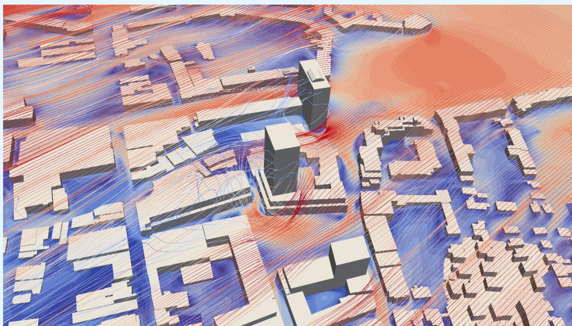
figuur 13: luchtstromingen vanuit zuidwestelijke richting rondom de hoge toren in het plangebied
