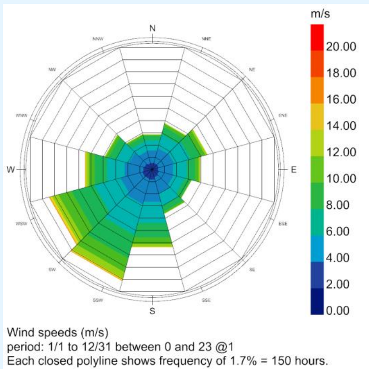
figuur 6: windstatistiek plangebied
