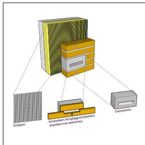
Figuur 23. Gebruik van een VMPM4 entreesteen (bron: faunaprojecten.nl).
