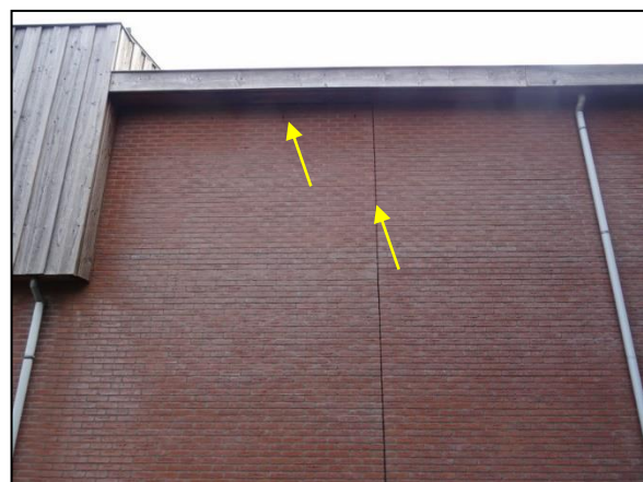
Figuur 12. Open stootvoegen en brede dilatatievoeg. Het linker deel van de muur blijft met de aanbouw ongewijzigd.
