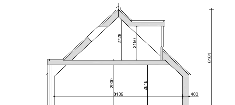
DOORSNEDE 2
