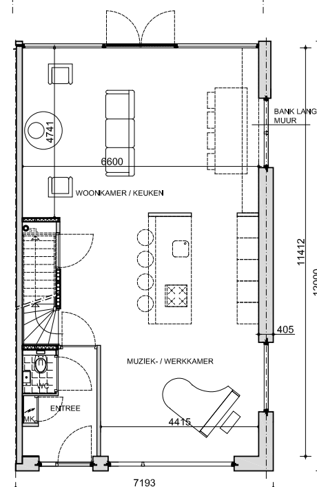
BEGANEGROND OPTIE 1
