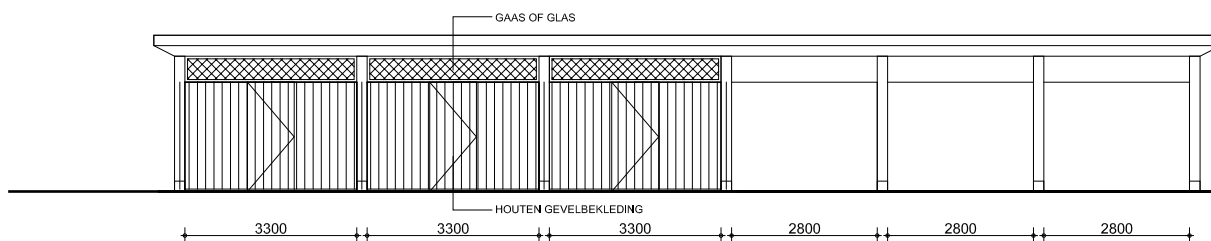
VOORAANZICHT
