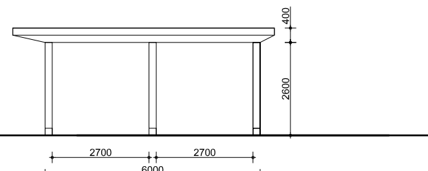
RECHTER ZIJAANZICHT
