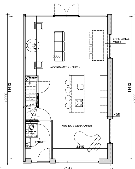
BEGANEGROND OPTIE 1
