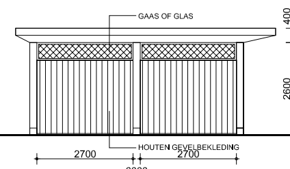
LINKER ZIJAANZICHT
