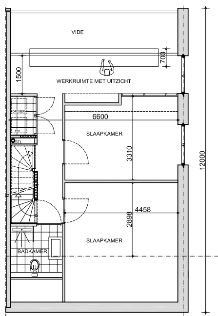
1E VERDIEPING 2E VERDIEPING = ZOLDER / EXTRA SLAAPKAMER
