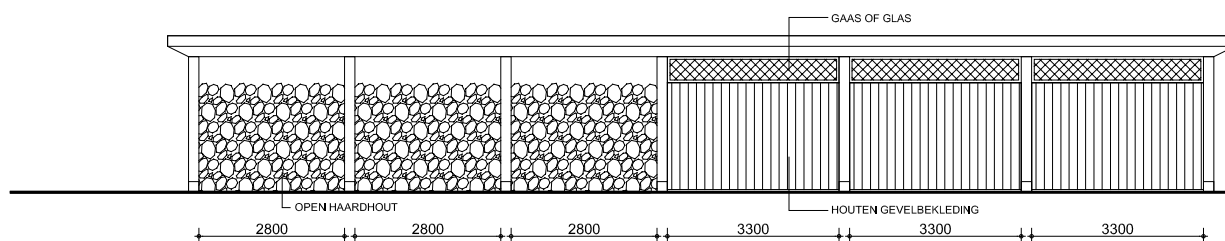
ACHTERAANZICHT
