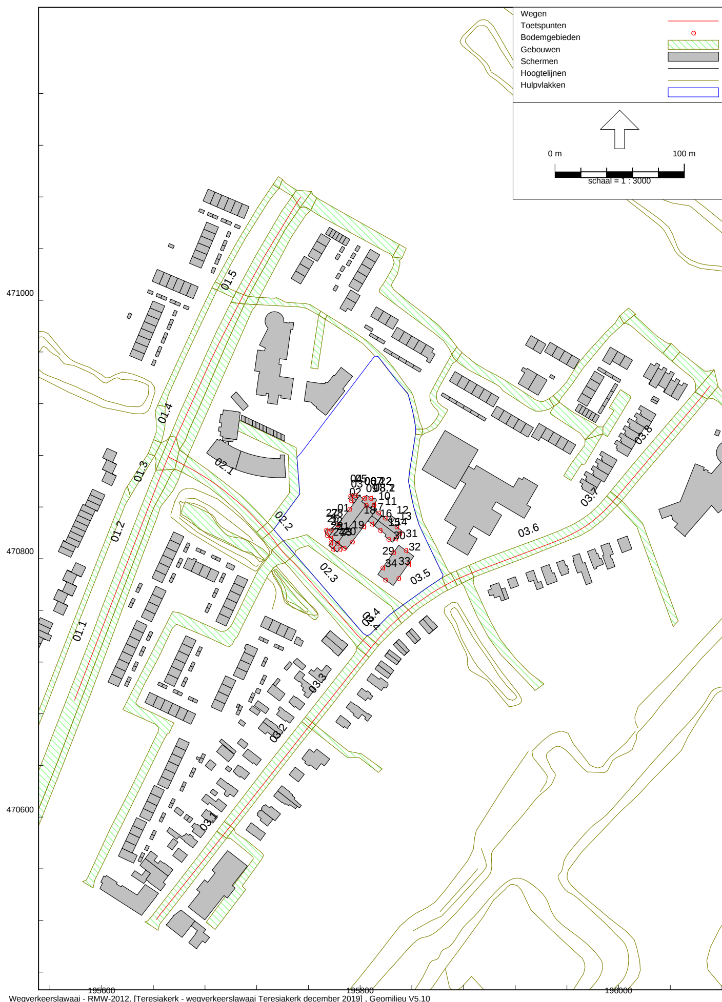
Overzicht van het rekenmodel met objecten, bodemgebieden, wegen en toetspunten
