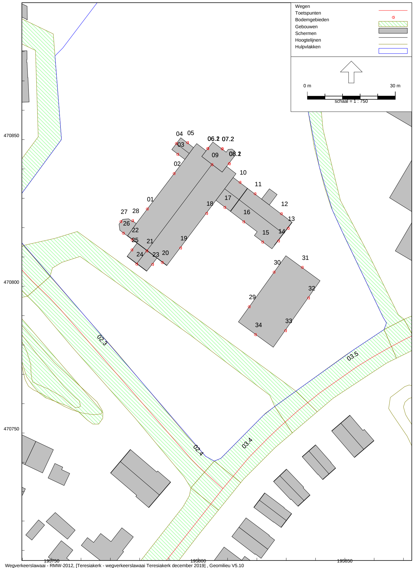
Detailoverzicht van het rekenmodel met objecten, bodemgebieden, wegen en toetspunten
