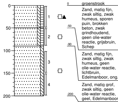
Boring: 2 boormeester R. Velderman Sleuflengte [m]: 0,30 Sleufbreedte [m]: 0,30
