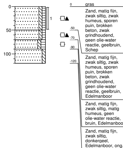
Boring: 5 boormeester R. Velderman Sleuflengte [m]: 0,30 Sleufbreedte [m]: 0,30
