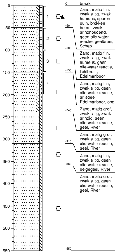
Boring: 1 boormeester R. Velderman Sleuflengte [m]: 0,30 Sleufbreedte [m]: 0,30
