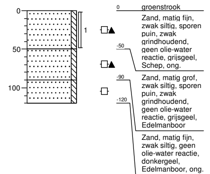
Boring: 6 boormeester R. Velderman Sleuflengte [m]: 0,30 Sleufbreedte [m]: 0,30
