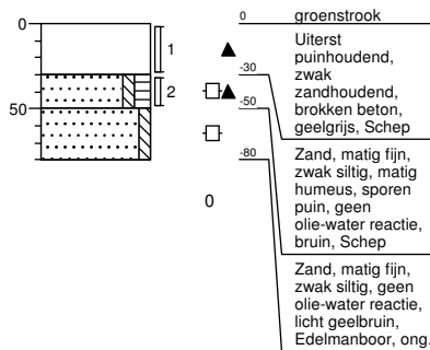
Boring: 4 boormeester R. Velderman Sleuflengte [m]: 0,30 Sleufbreedte [m]: 0,30
