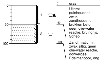
Boring: 10 boormeester R. Velderman Sleuflengte [m]: 0,30 Sleufbreedte [m]: 0,30
