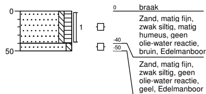
Boring: 11 boormeester R. Velderman Sleuflengte [m]: 0,00 Sleufbreedte [m]: 0,00
