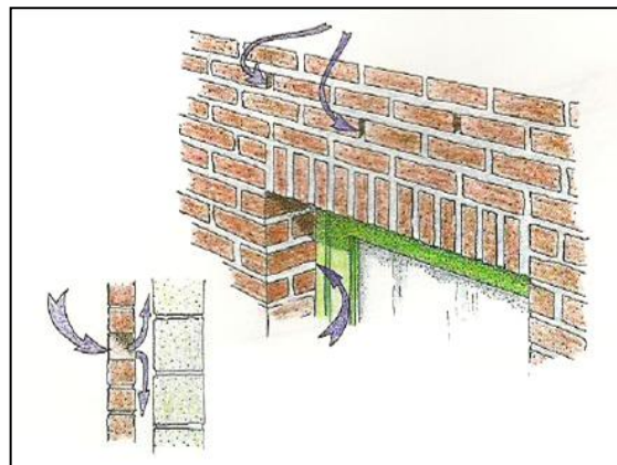
Figuur 12. Voorbeeld toegang tot de luchtspouw is een eenvoudige maatregel om nieuwbouw geschikt te maken (bron: vleermuizeninfo.be).
