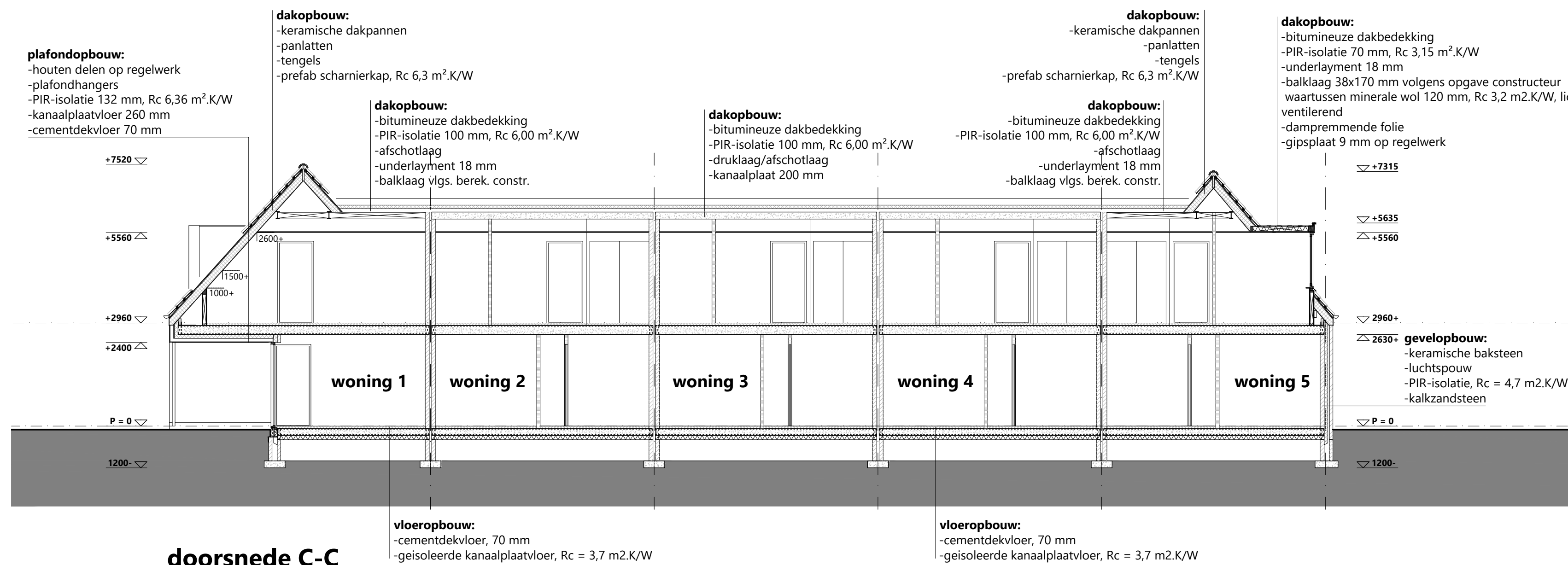
doorsnede C-C
