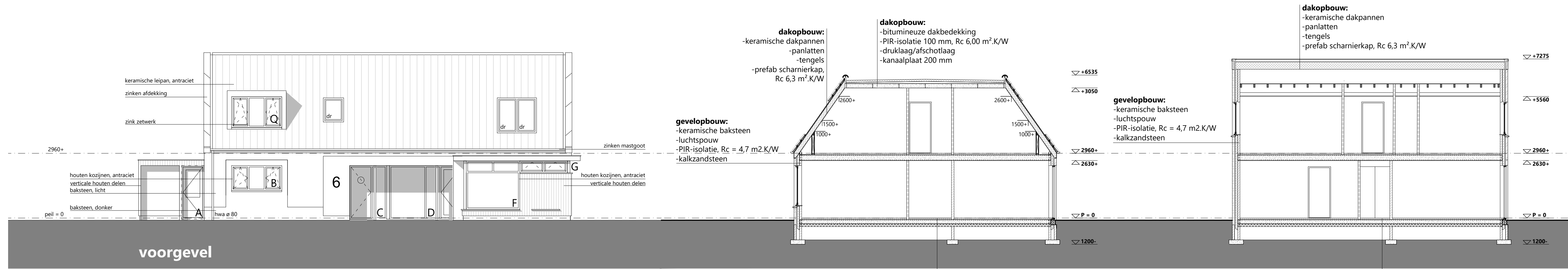
doorsnede A-A
