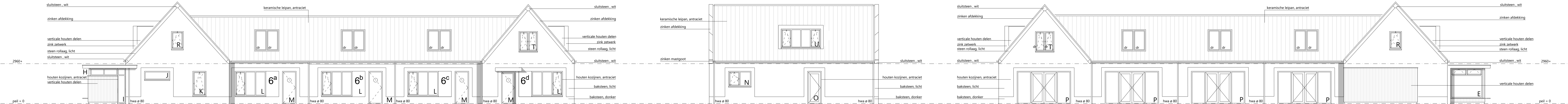
rechter zijgevel achtergevel linker zijgevel
