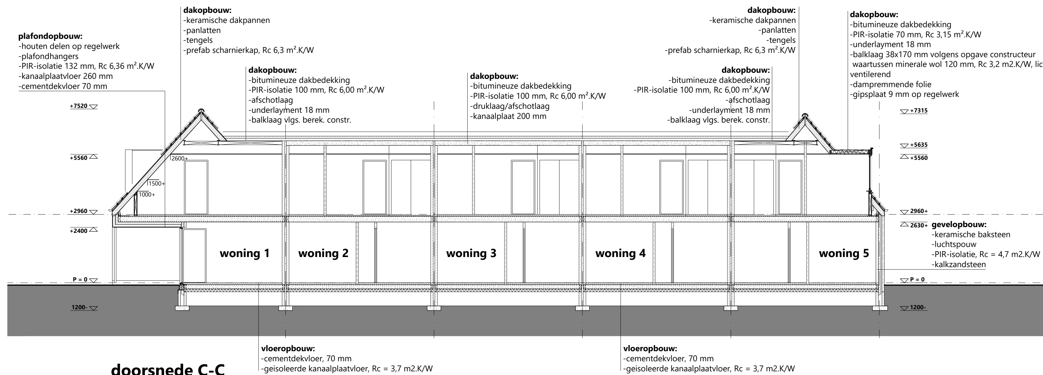
doorsnede C-C
