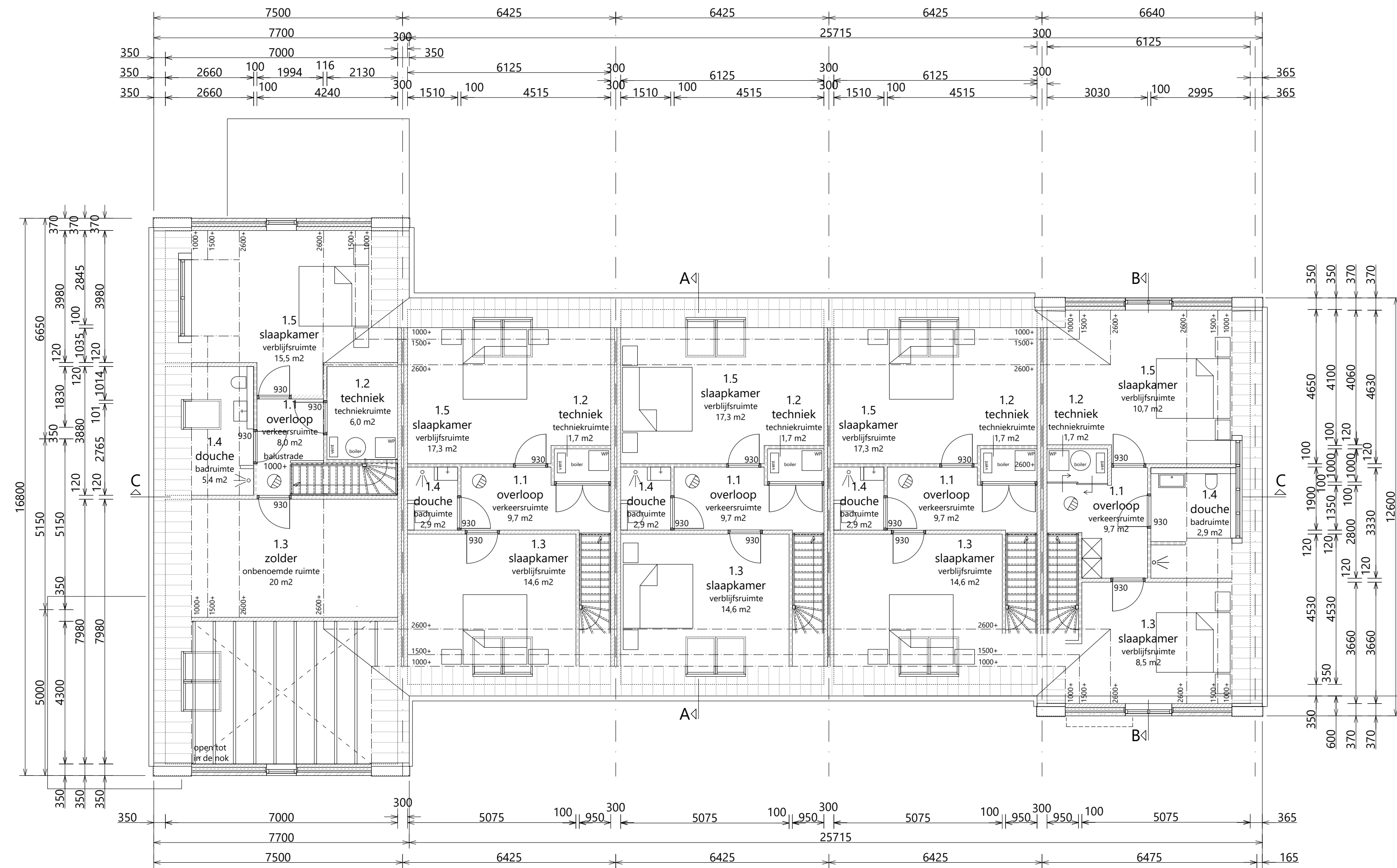
1e verdieping
