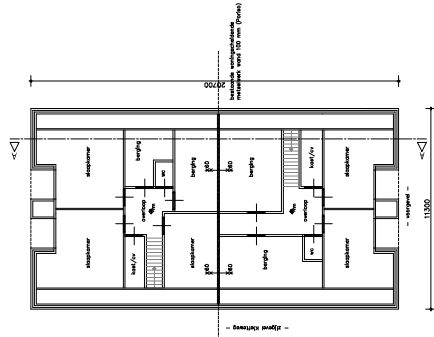
1e verdieping
