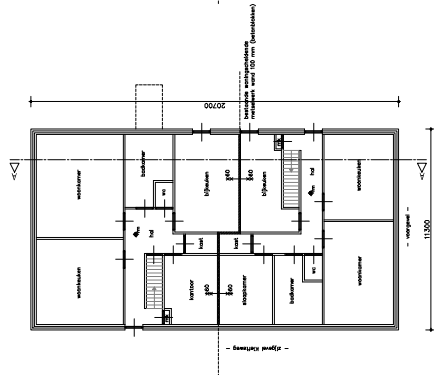
begane grond
