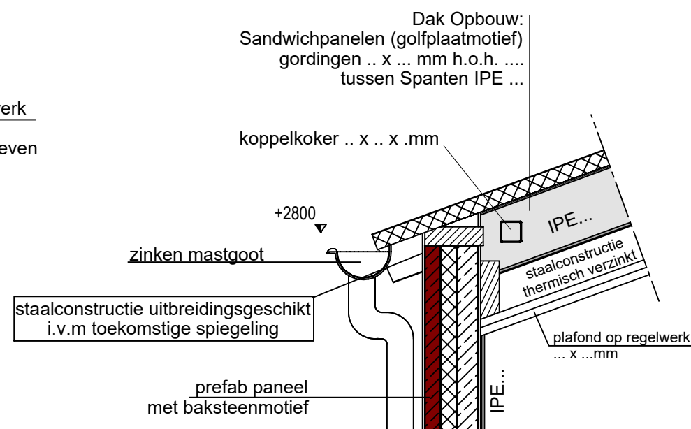
2. Principe detail zijgevel
