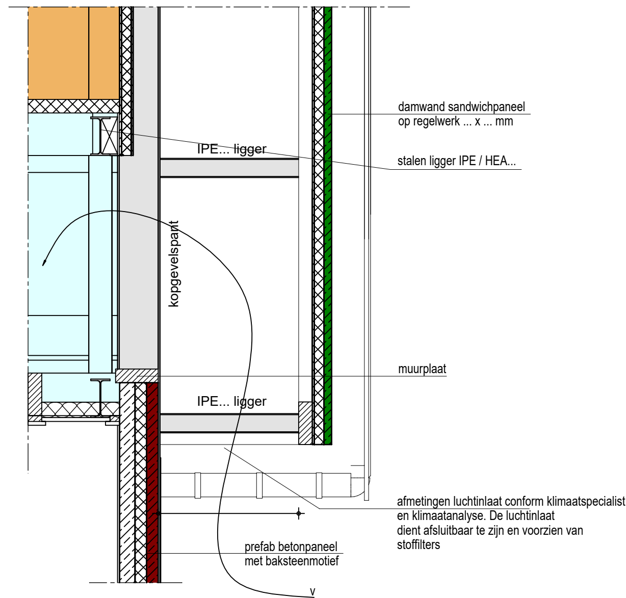
4.Principe detail kopgevel
