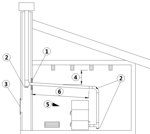
Fig. 13 - Voorbeeld 2
