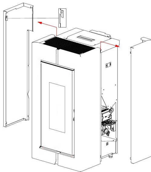
Fig. 28 - De zijpanelen losmaken
