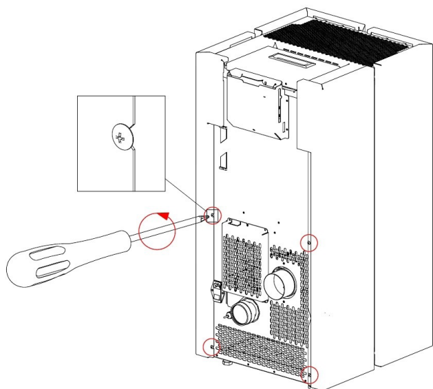
Fig. 27 - Verwijder de schroeven
