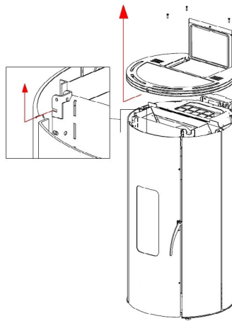
Fig. 38 - Verwijdering van de afdekking
