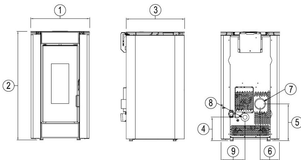
Fig. 16 - Algemene afmetingen: Evo³
