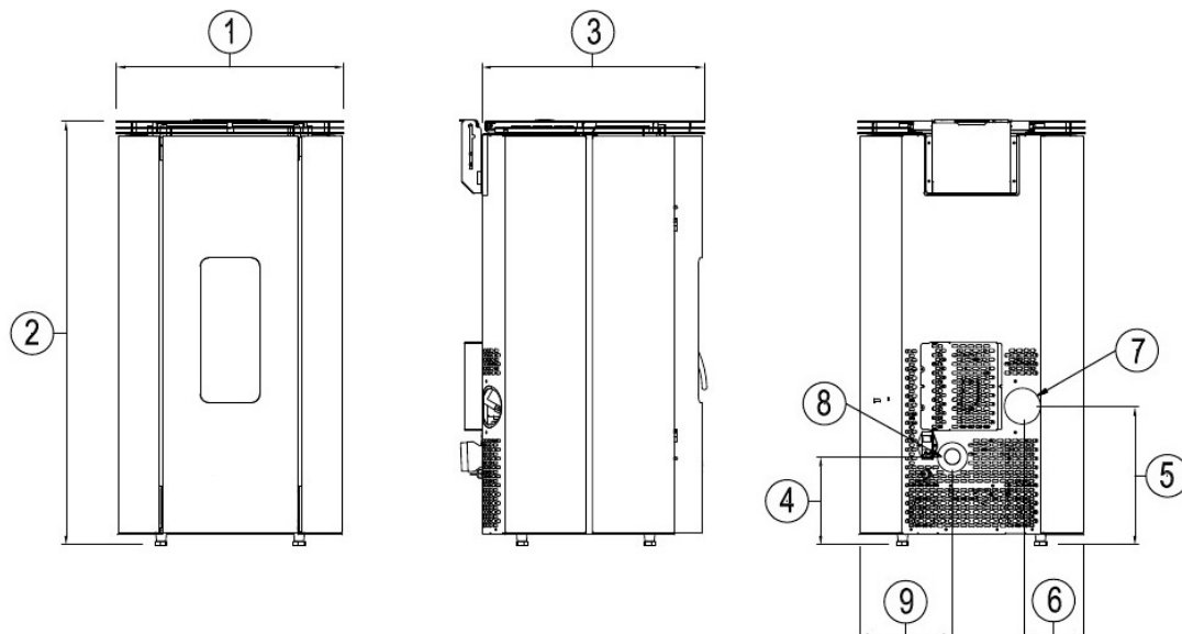
Fig. 19 - Algemene afmetingen: Shell³
