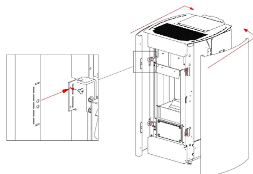
Fig. 33 - Verwijdering zijpanelen
