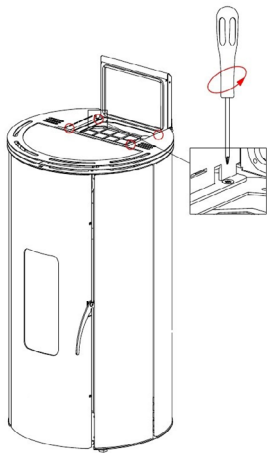
Fig. 37 - Verwijder de schroeven
