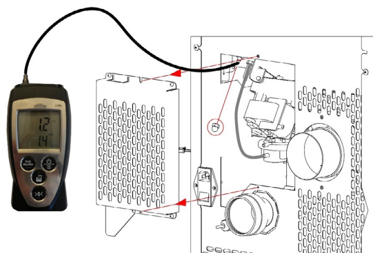
Fig. 55 - Aansluiting digitale drukregelaar
