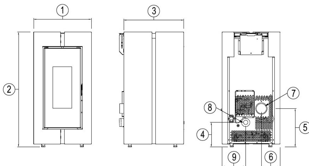
Fig. 15 - Algemene afmetingen: Tecna³
