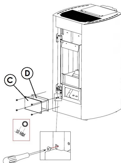
Fig. 68 - Verwijdering van de plaat
