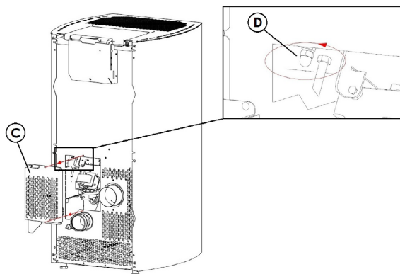
Fig. 54 - Carter verwijderen
