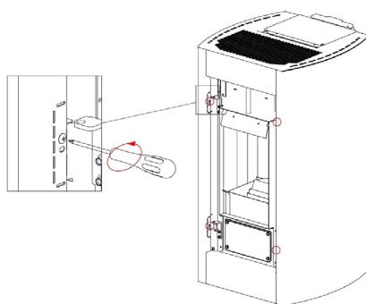
Fig. 32 - Verwijder de schroeven
