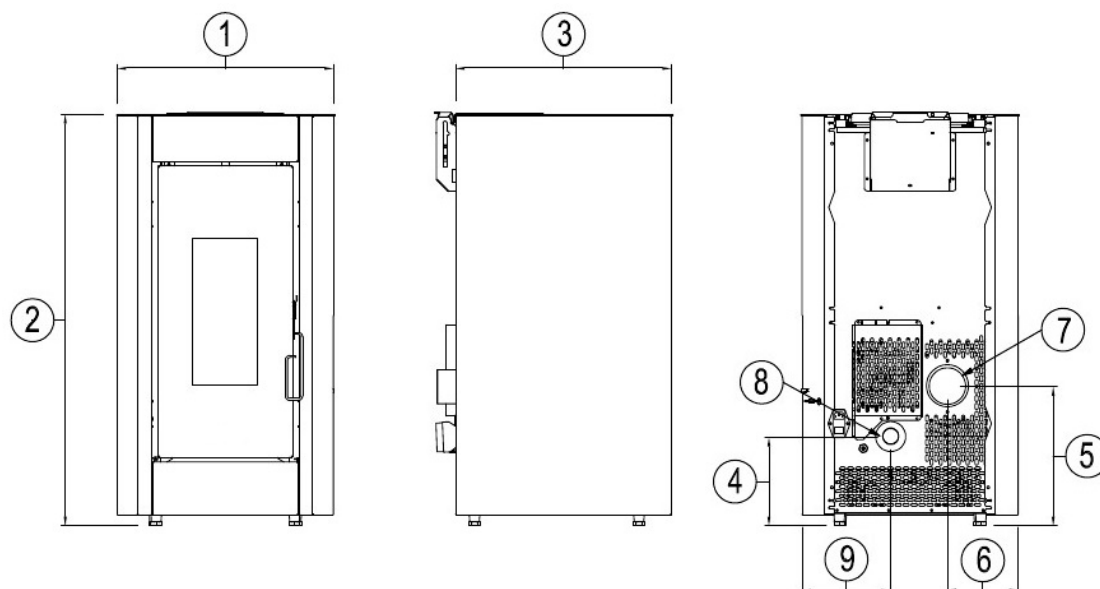
Fig. 17 - Algemene afmetingen: Kriss³
