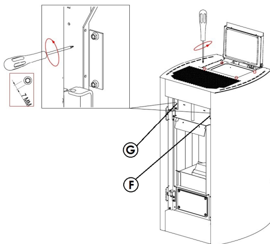
Fig. 66 - Verwijdering van de platen
