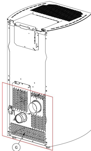
Fig. 70 - Achterste rooster
