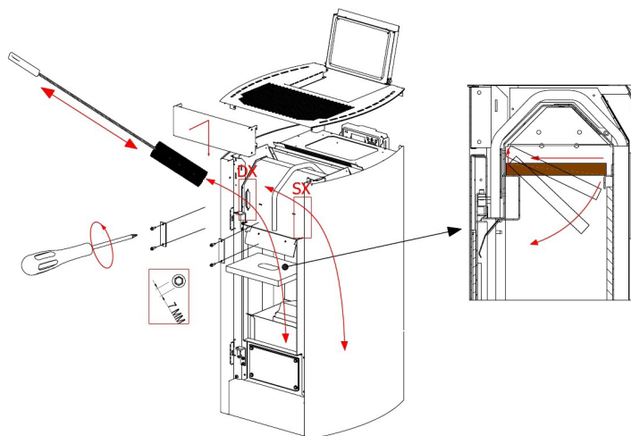
Fig. 67 - Reiniging
