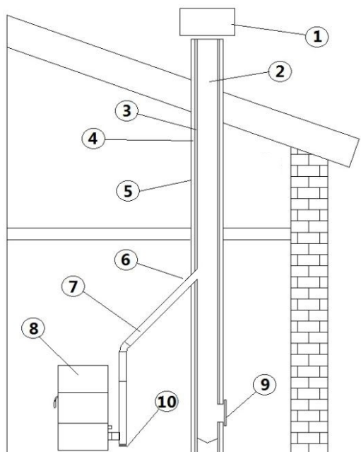
Fig. 5 - Onderdelen van de schoorsteen
