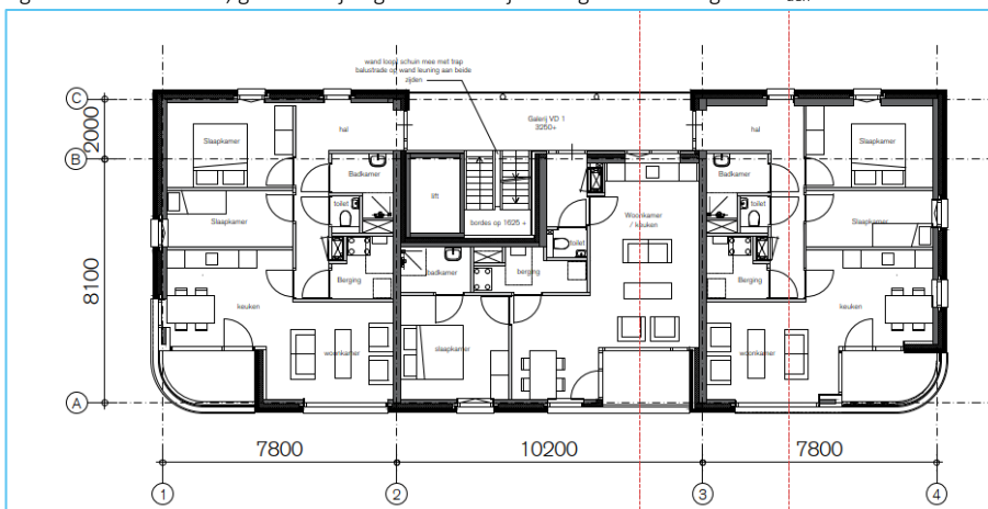
Figuur 23: Woningindeling bouwdeel 6
