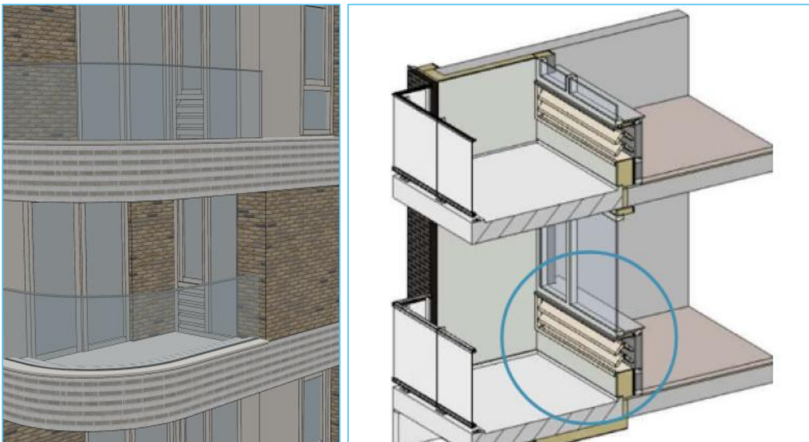
Figuur 16: Twee voorbeelden van een laag spuisysteem achter dichte balkonbalustrade
