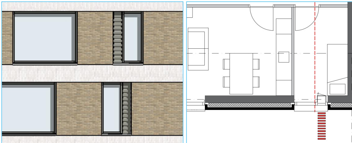
Figuur 17: Aanzicht en plattegrond van geluiddempend rooster in de slaapkamer.
