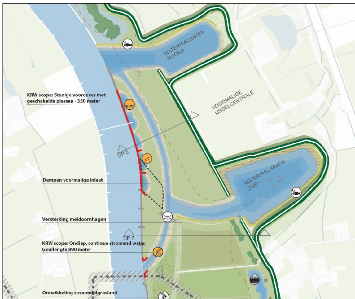
Figuur 3-7 Indicatieve ligging meestromende nevengeul en natuurlijke oevers (Schetsontwerp oktober 2023, GROW).
