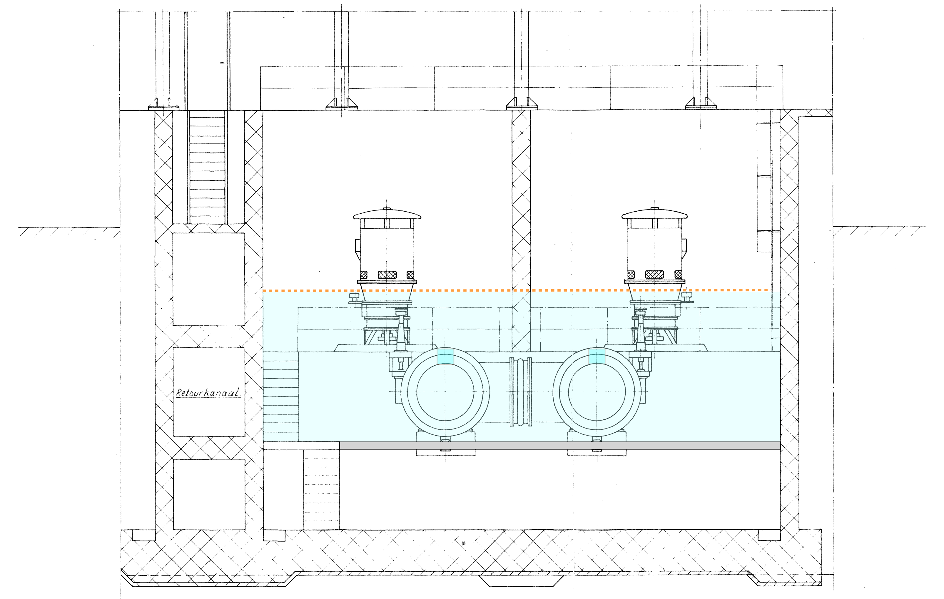
Doorsnede A-A
