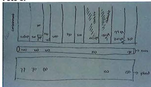
Schets wand met meetwaarden
