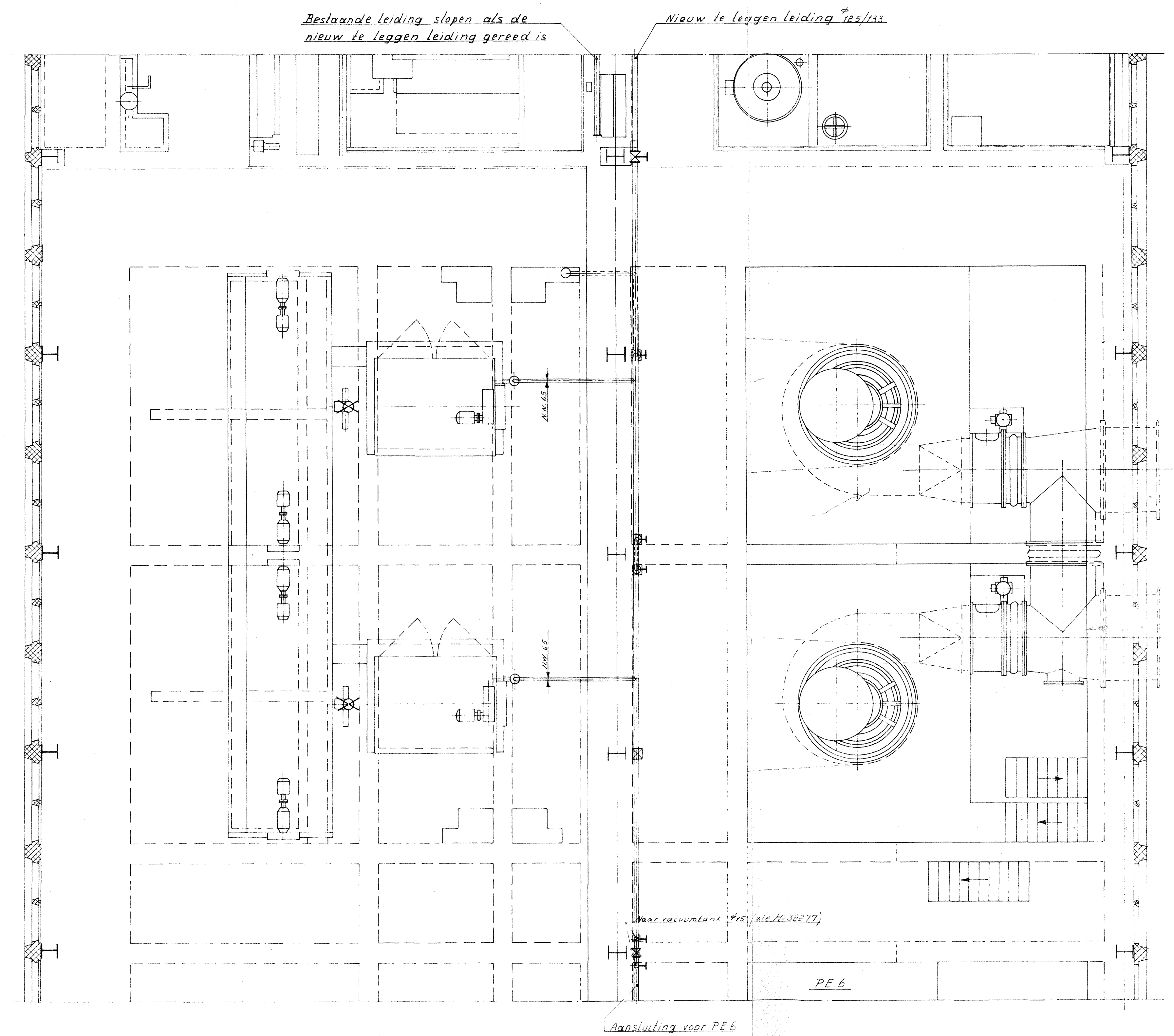
Overzicht vloer 5200
