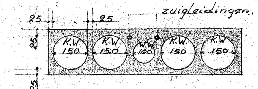
Doorsnede C-C
