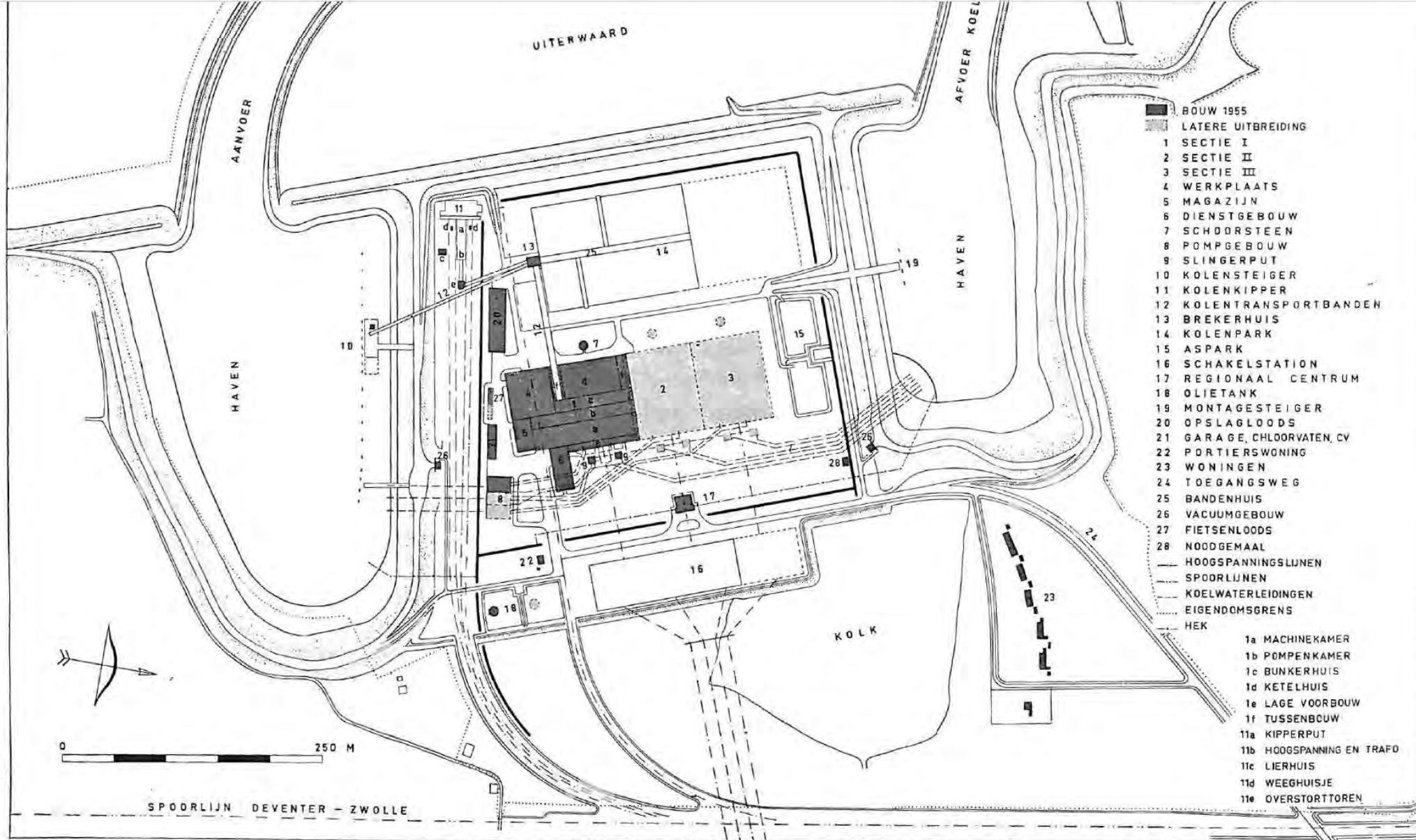
situatietekening 1955
