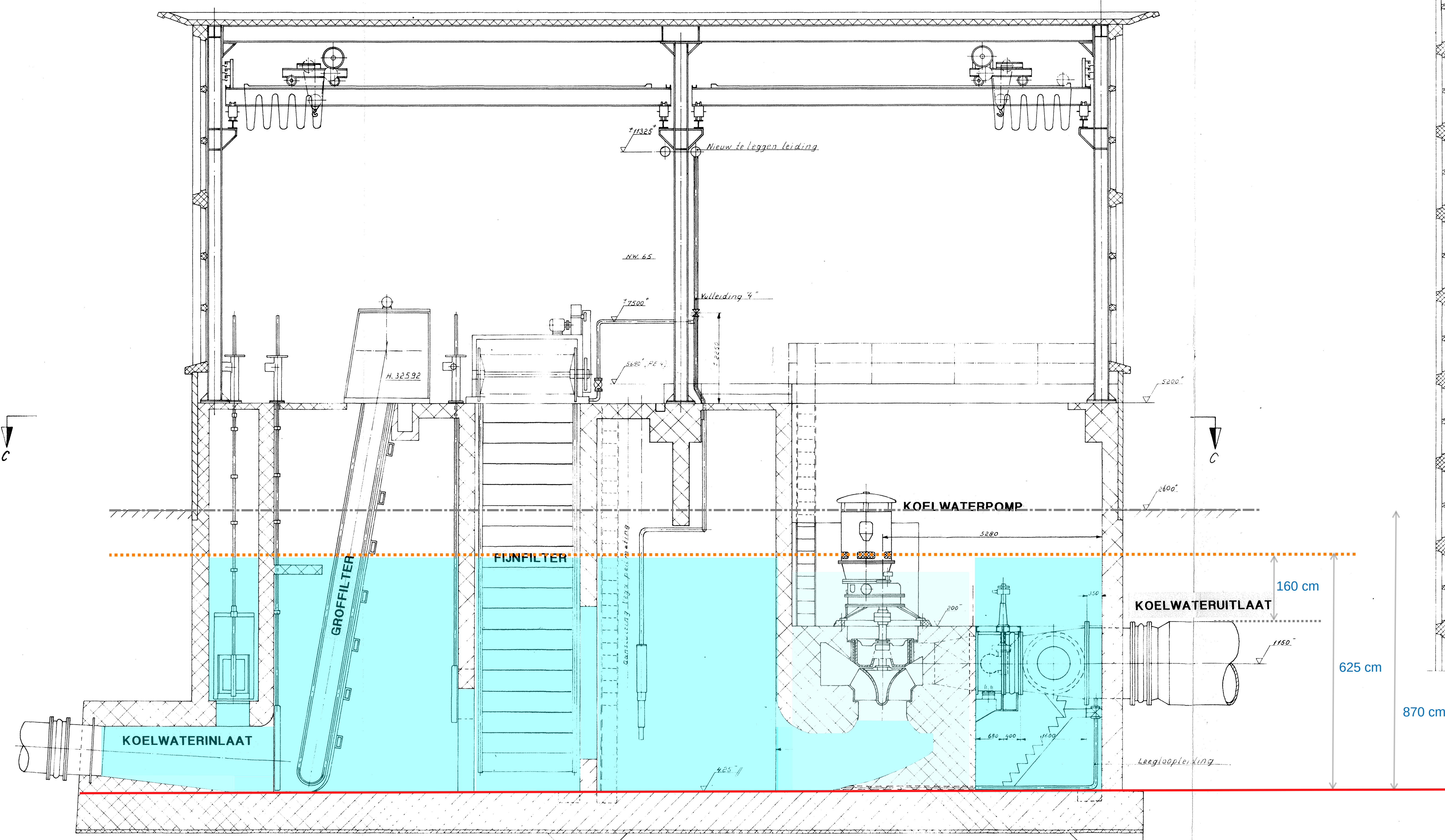
Doorsnede B-B
