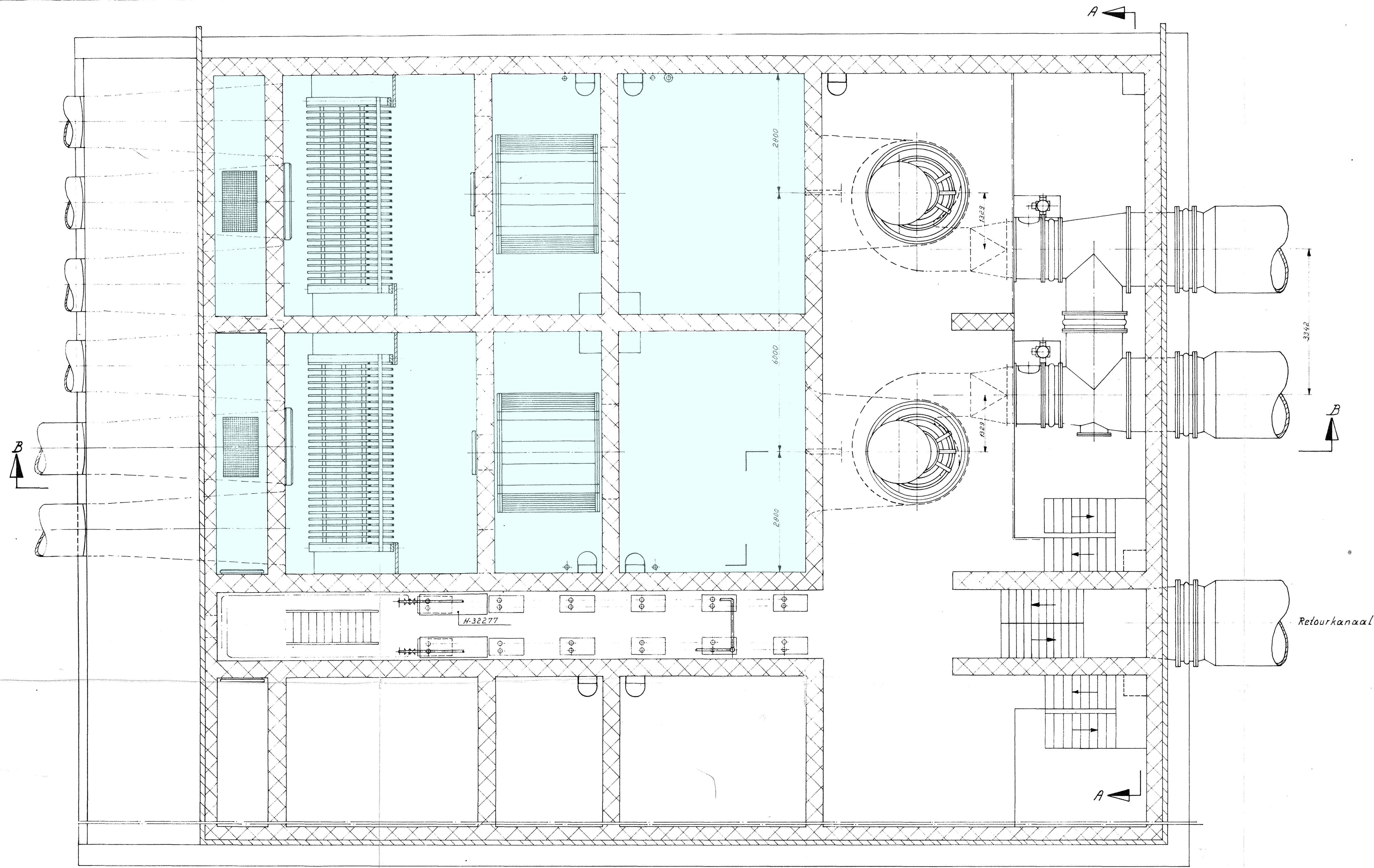
Doorsnede C-C
