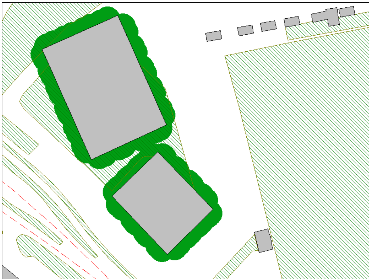
Figuur 4.5: Geluidbelasting t.g.v. wegverkeer op de A28 (incl. aftrek art. 110g Wgh)
