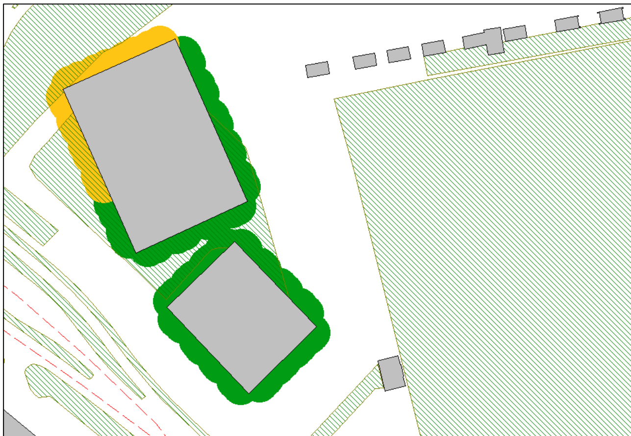
Figuur 4.3: Geluidbelasting t.g.v. wegverkeer op de Van Wevelinkhovenstraat (incl. aftrek art. 110g Wgh)
