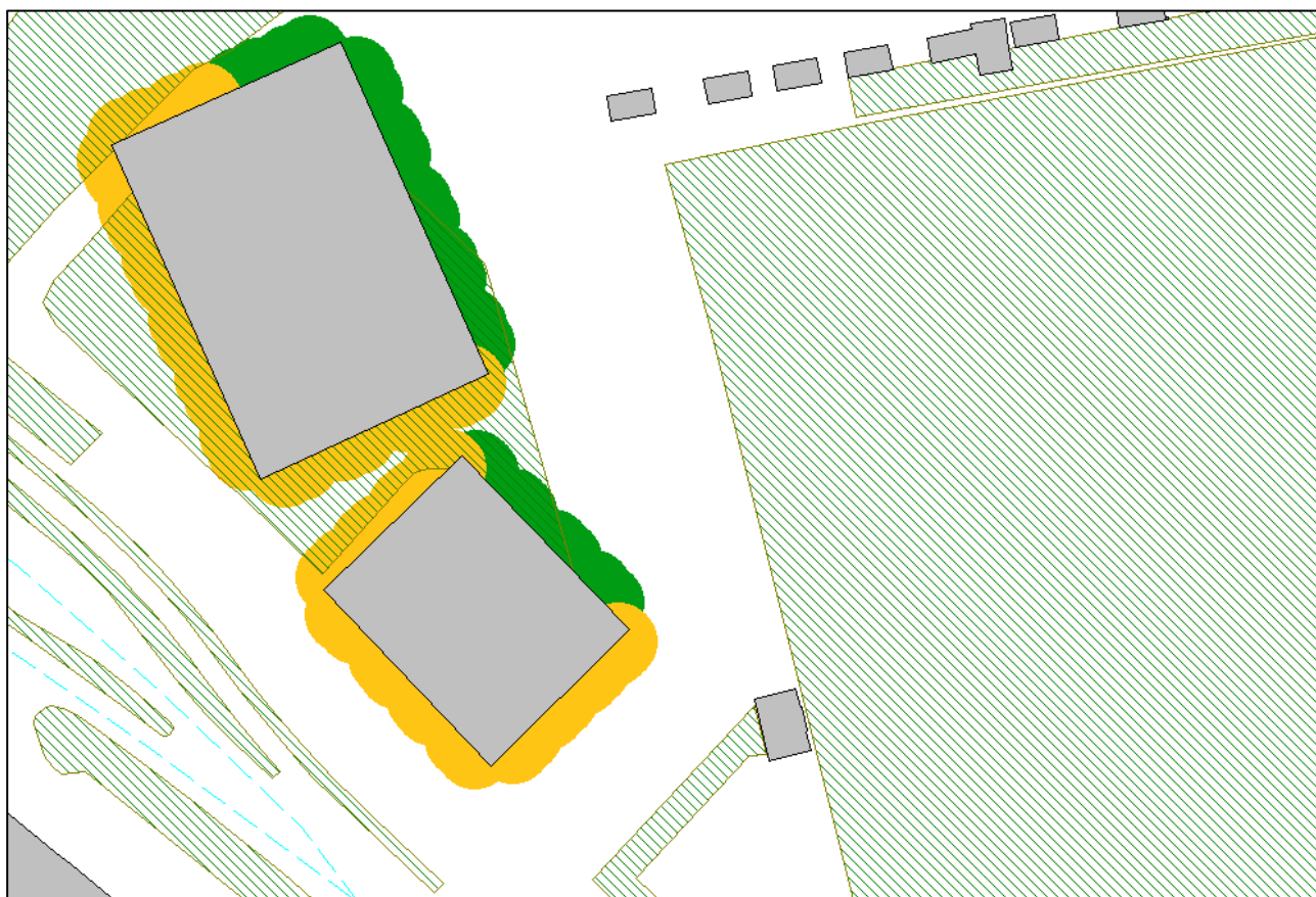
Figuur 4.2: Geluidbelasting t.g.v. wegverkeer op de Bisschop Wildebrandlaan en Middelweg (incl. aftrek art. 110g Wgh)
