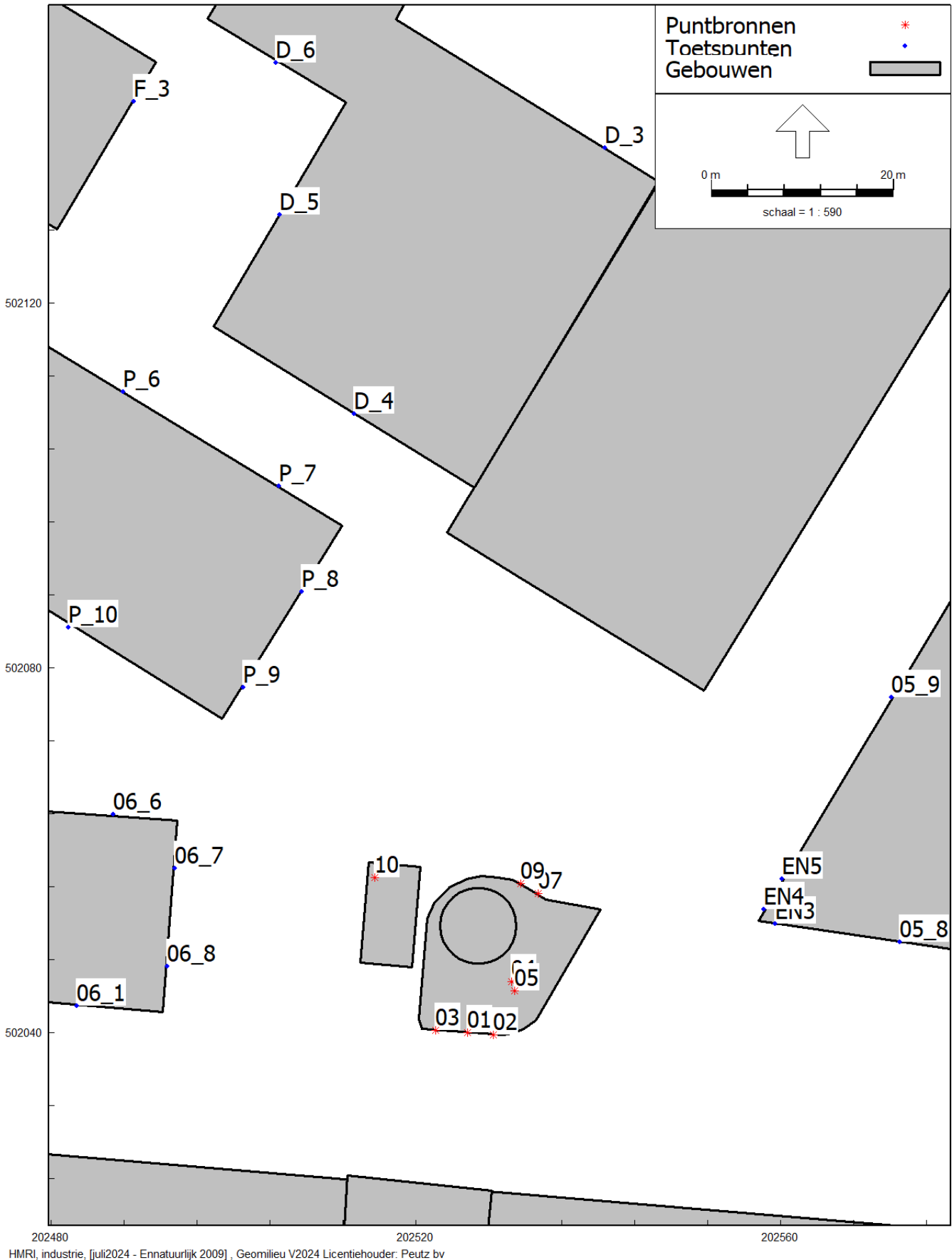
Weergave rekenmodel
