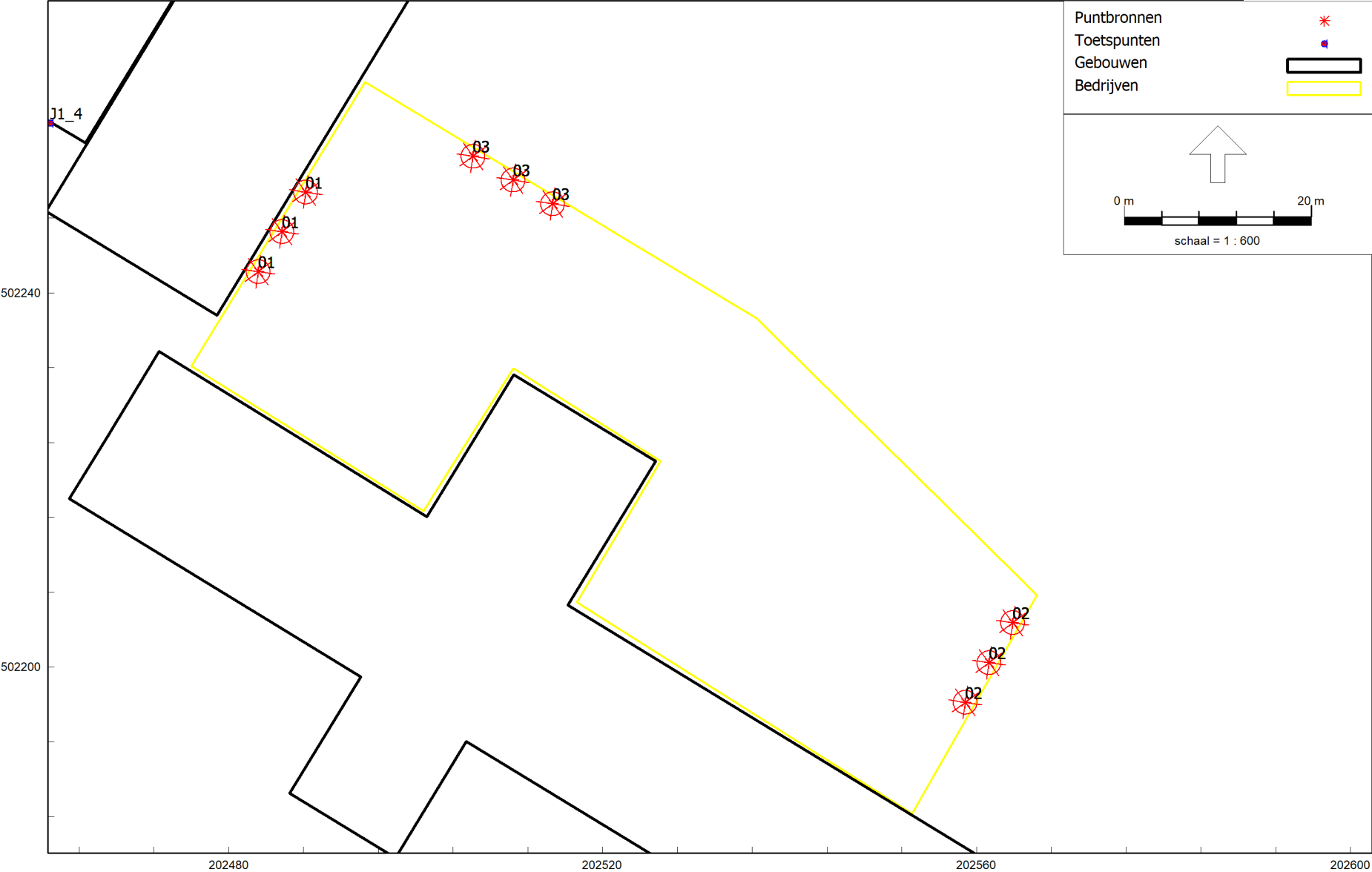
Schematische weergave rekenmodel Evenementenlocatie 3 Spoorpark perron 038
