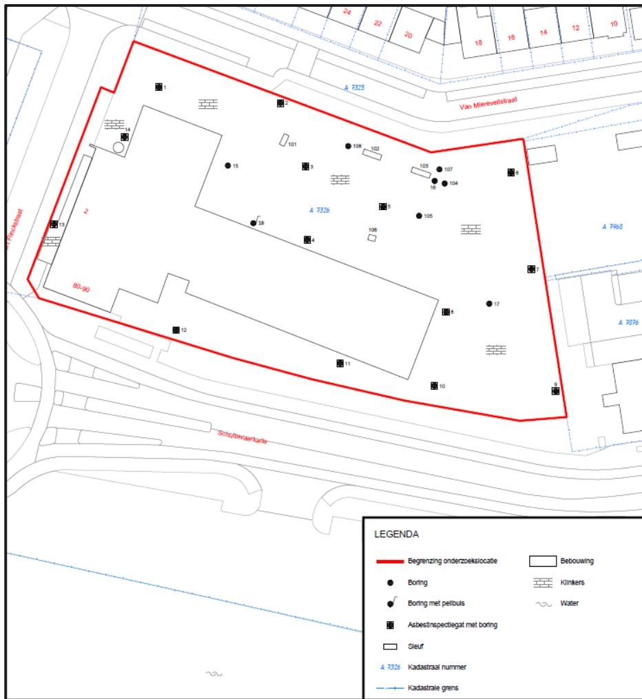
Figuur 19: Situatietekening onderzoekslocatie met geplaatste boringen
