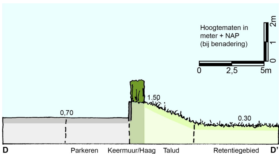
Afbeelding: Doorsnede D - D'
