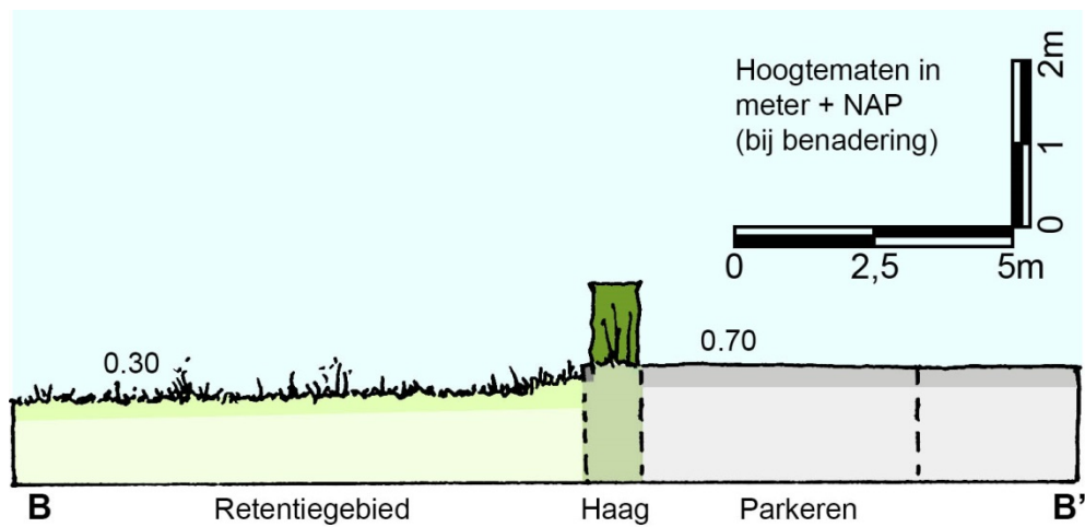
Afbeelding: Doorsnede B - B'
