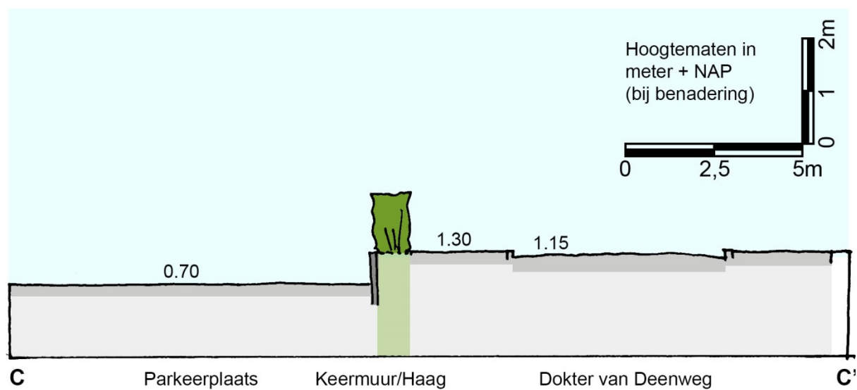
Afbeelding: Doorsnede C - C'
