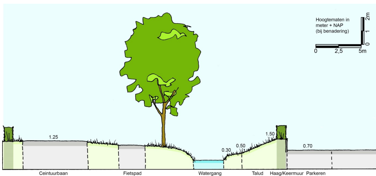
Afbeelding: Doorsnede A - A'
