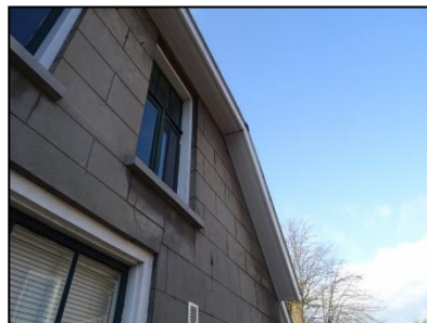
Figuur 14. Geen ruimtes onder tussen de aftimmering en de muur. Daarnaast zijn er geen open stootvoegen aanwezig.
