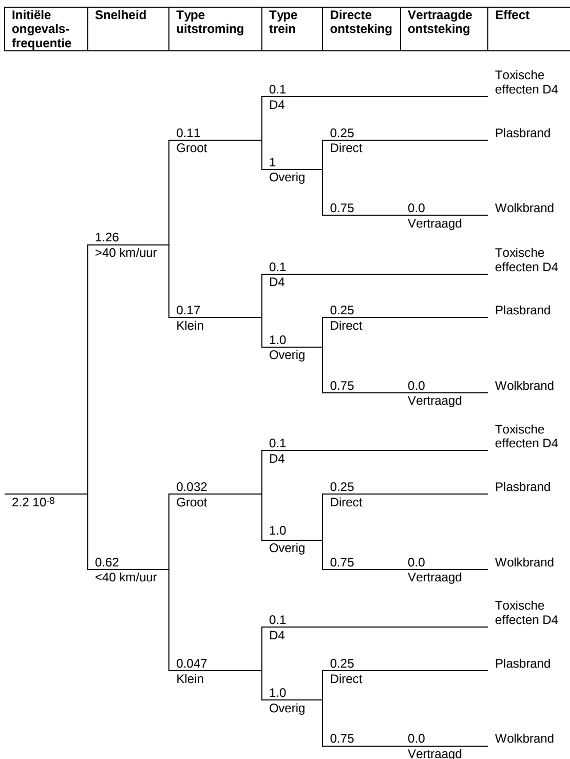
Figuur 1.2. RBM II gebeurtenisboom uitstroming brandbare vloeistof uit spoorketelwagen
