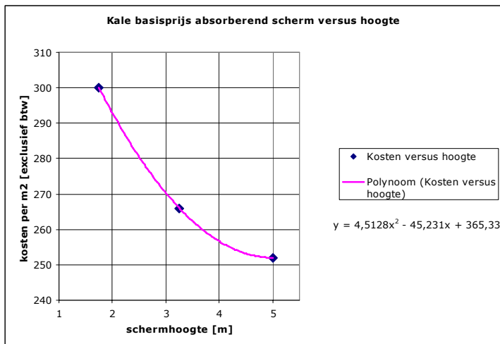
Figuur 9: Trendlijn schermkosten
