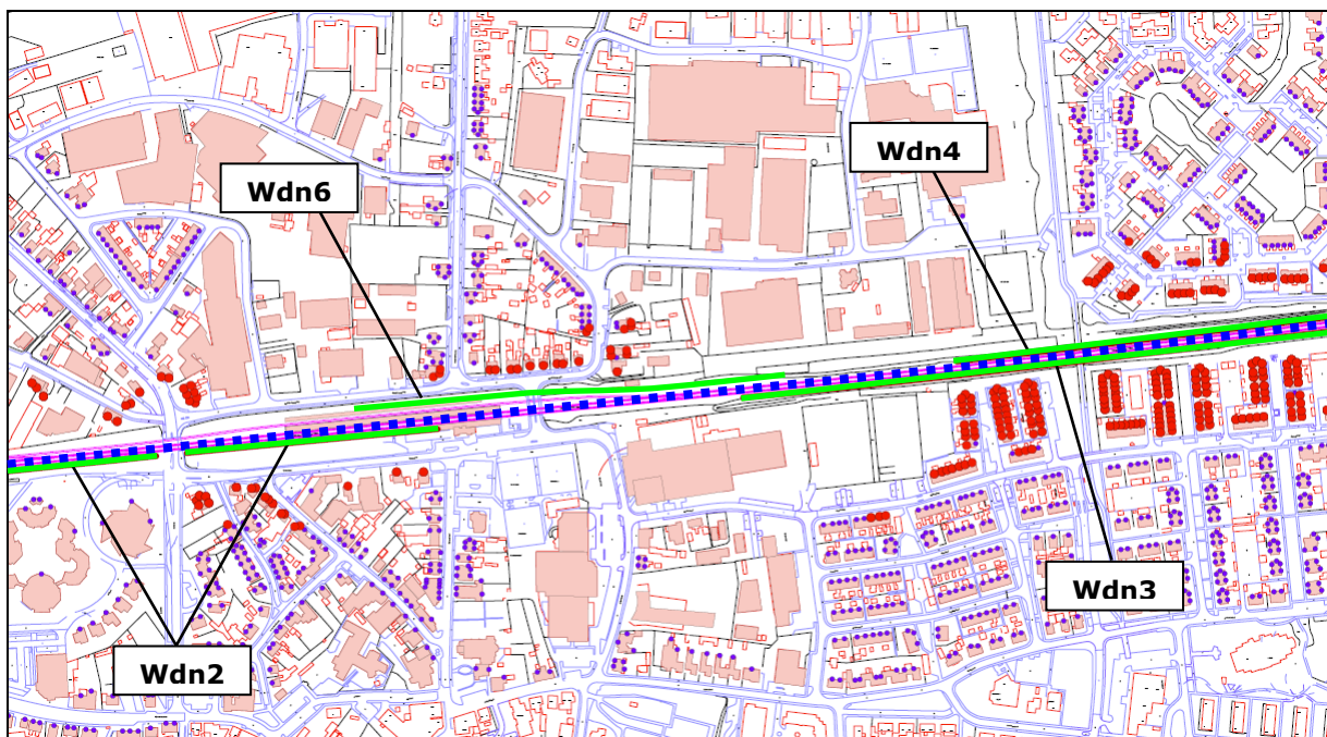
Figuur 12: Saneringswoningen, raildempers en schermplaatsing Wdn2-oost, Wdn3-west, Wdn4-west en Wdn6
