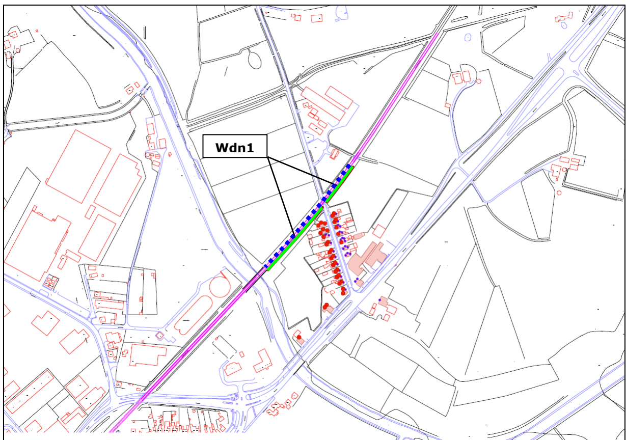
Figuur 10: Saneringswoningen, raildempers en schermplaatsing Wdn1 (nabij Klokkendijk)
