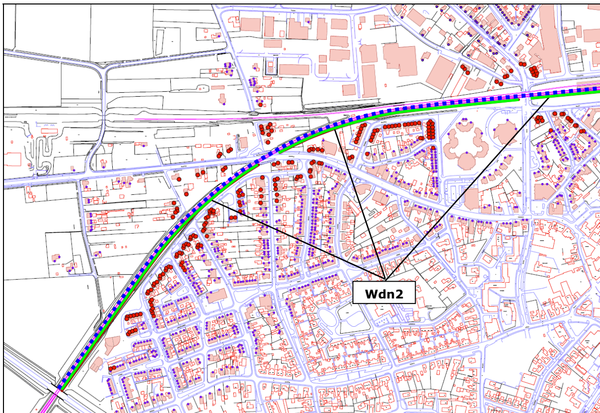
Figuur 11: Saneringswoningen, raildempers en schermplaatsing Wdn2-west
