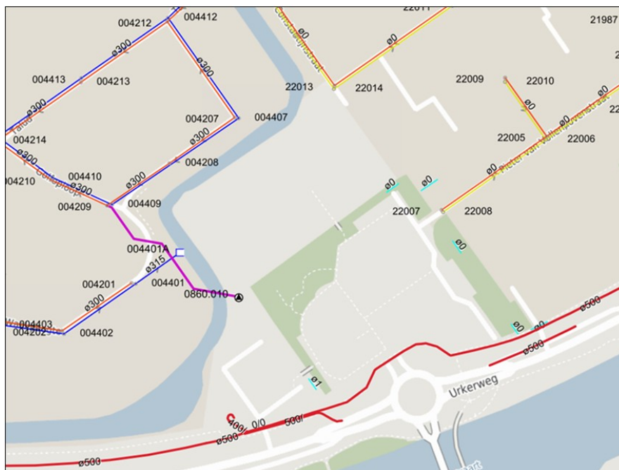
Rioolsysteem projectlocatie
