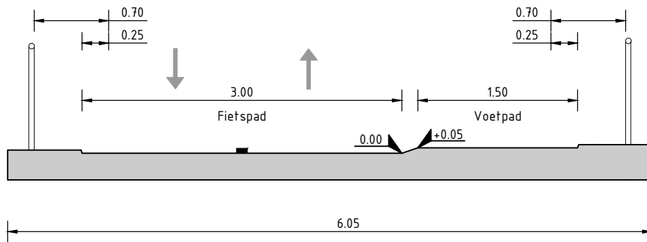
Principe-doorsnede nieuwe fiets-/loopbrug schaal 1:50
