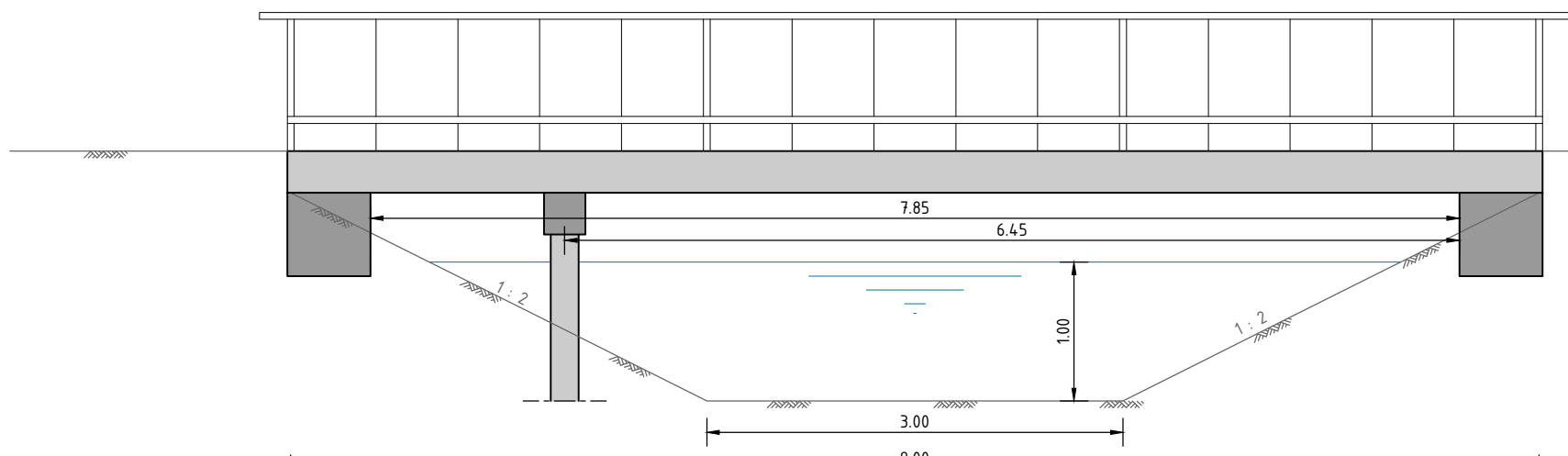
Principe-zijaanzicht nieuwe fiets-/loopbrug schaal 1:50
