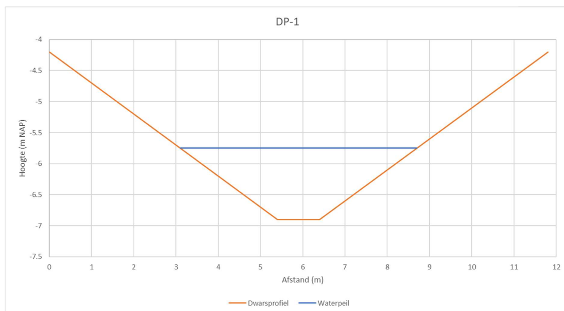
Figuur 7. Dwarsprofiel 1 (paarse watergang).
