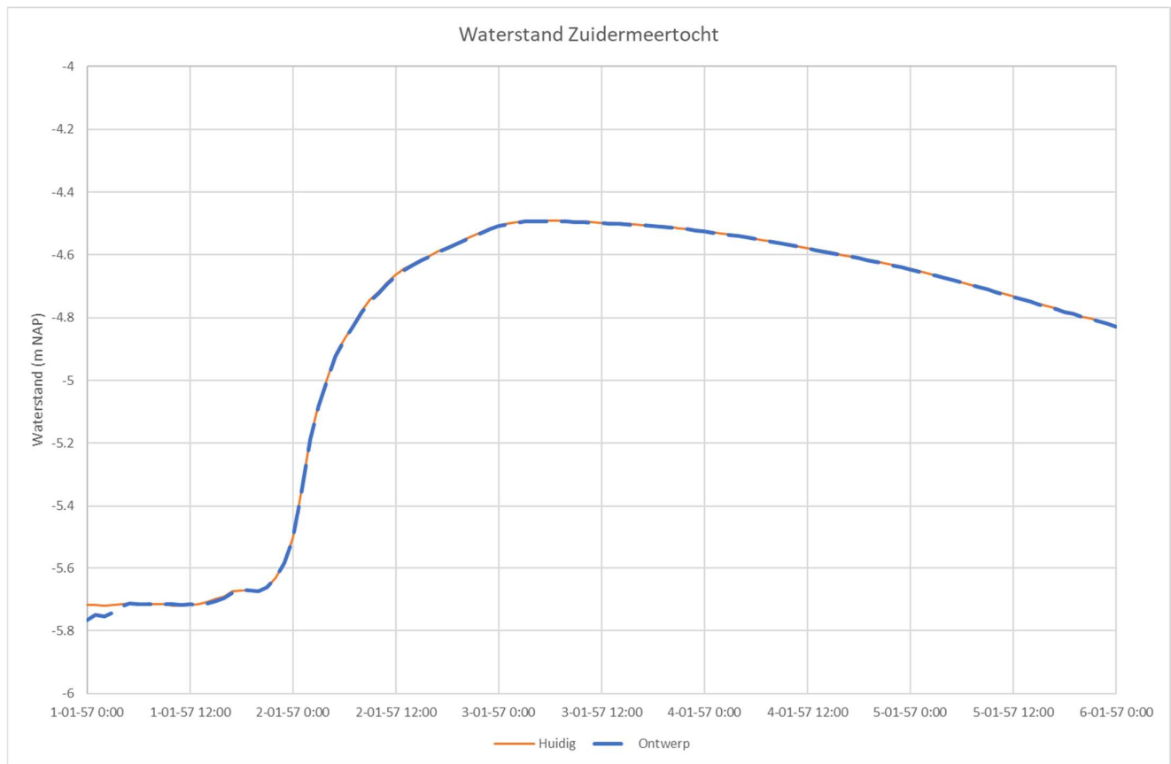
Figuur 5. Berekende waterstand in de Zuidermeertoicht bij zowel de huidige als toekomstige situatie.
