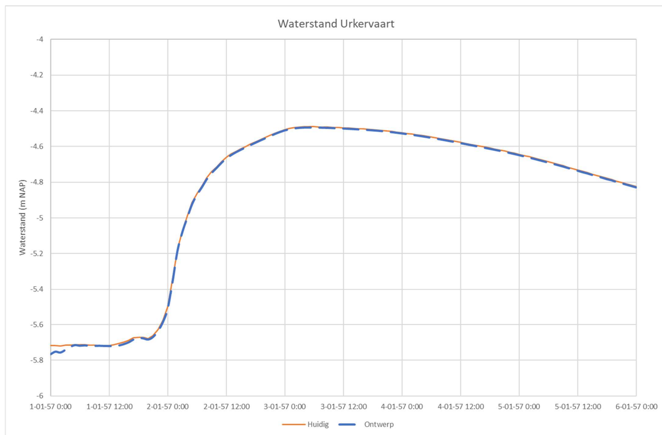
Figuur 4. Berekende waterstand in de Urkervaart bij zowel de huidige als ontwerp situatie.
