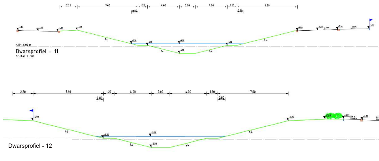
Figuur 9. Dwarsprofielen 11 en 12. Dit zijn de dwarsprofielen van de oost-west watergang.
