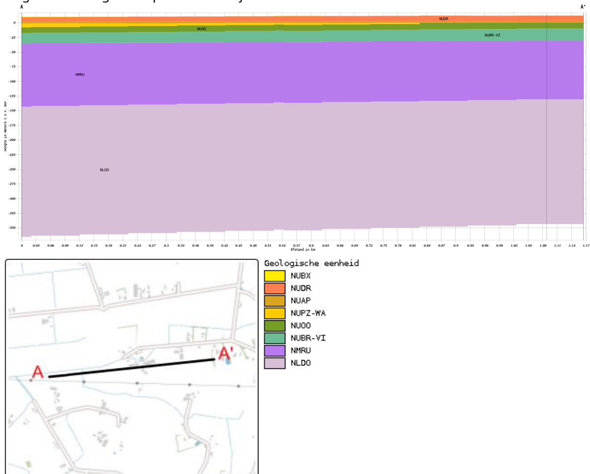
Figuur 1 Geologische opbouw landelijk model DGM v2.2
