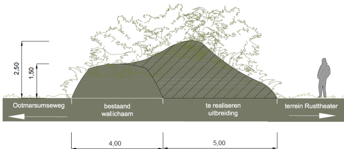
Figuur 3.2 Schematische weergaven dwarsprofiel wallichaam
