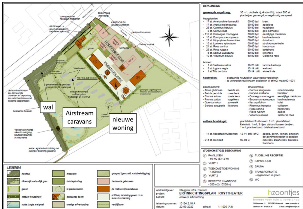
Figuur 3.1 Inrichtingsplan.
