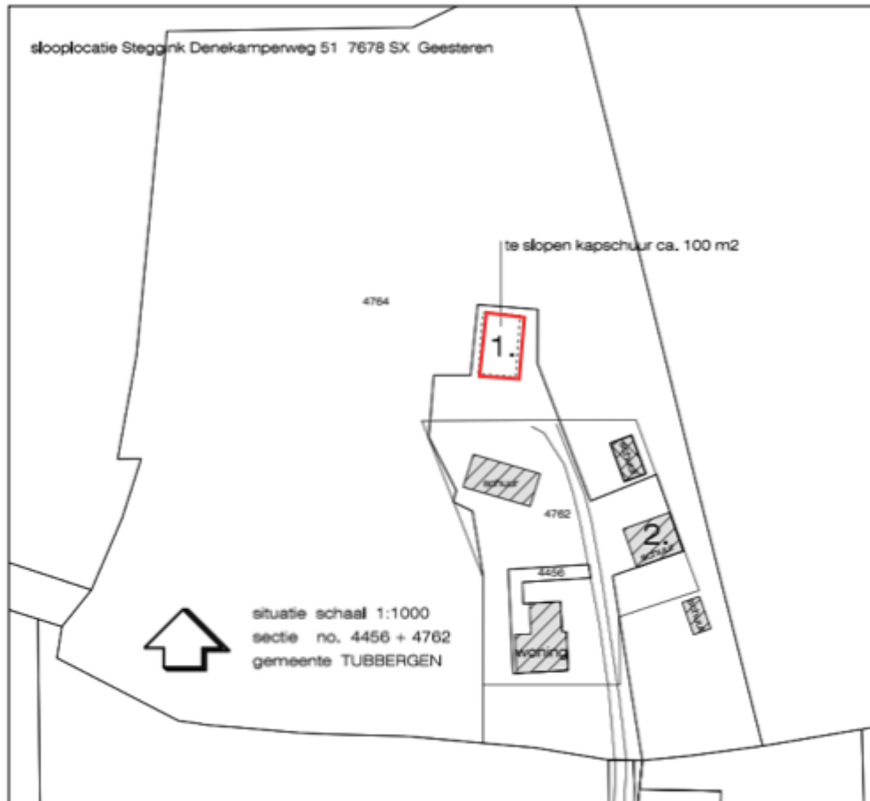
Afbeelding 3.1 Gewenste situatie Denekamperweg 51 (Bron: Erwin Meinders bouwkundig buro)
