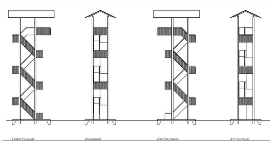
Aanzicht van de te bouwen uitkijktoren (bron: B+O Architectuur en interieur BV).
